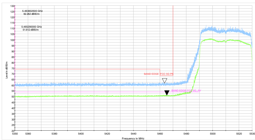
be40 CH102_5.35-5.53GHz_TP14
