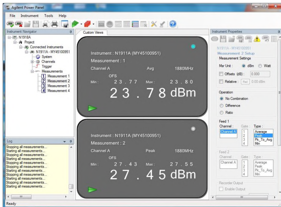
CA_2A-5A_10+10 MHz Bandwidth_1880 MHz 1-49 RB & 829 MHz 1-0 RB_QPSK
