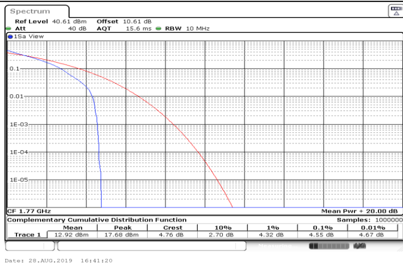
Band66-20MHz-QPSK-132572-100RB#0
