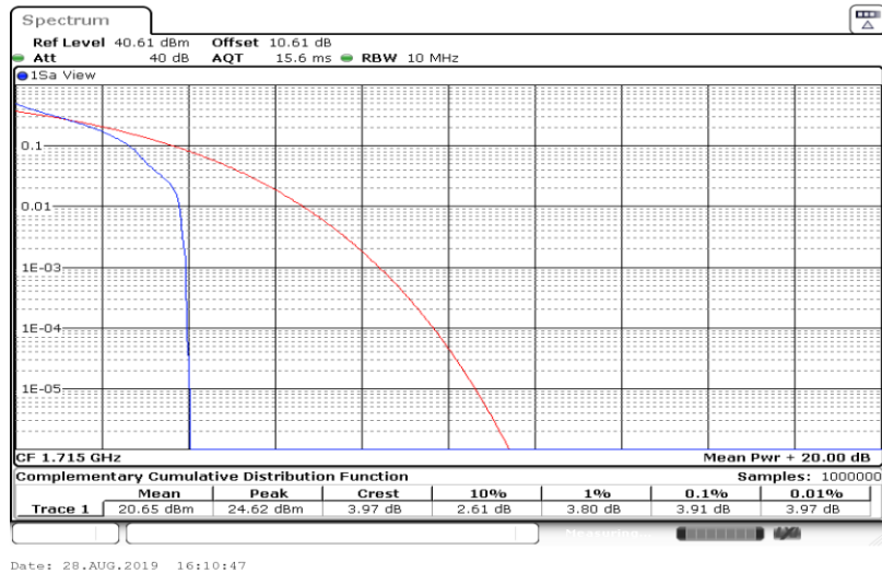
Band66-10MHz-QPSK-132022-50RB#0
