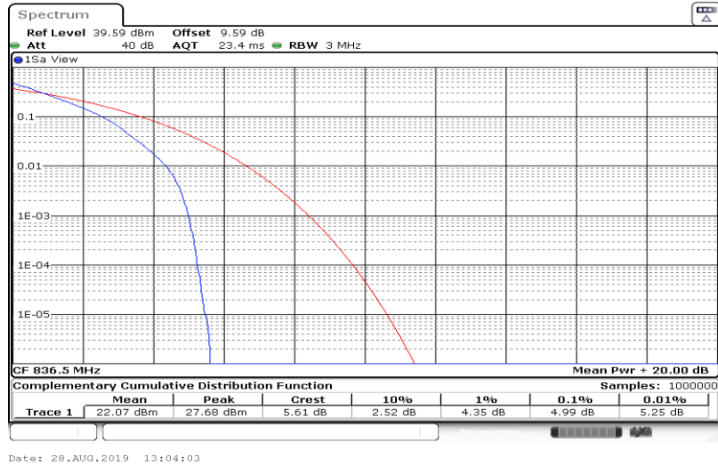
Band5-3MHz-QPSK-20635-1RB#0
