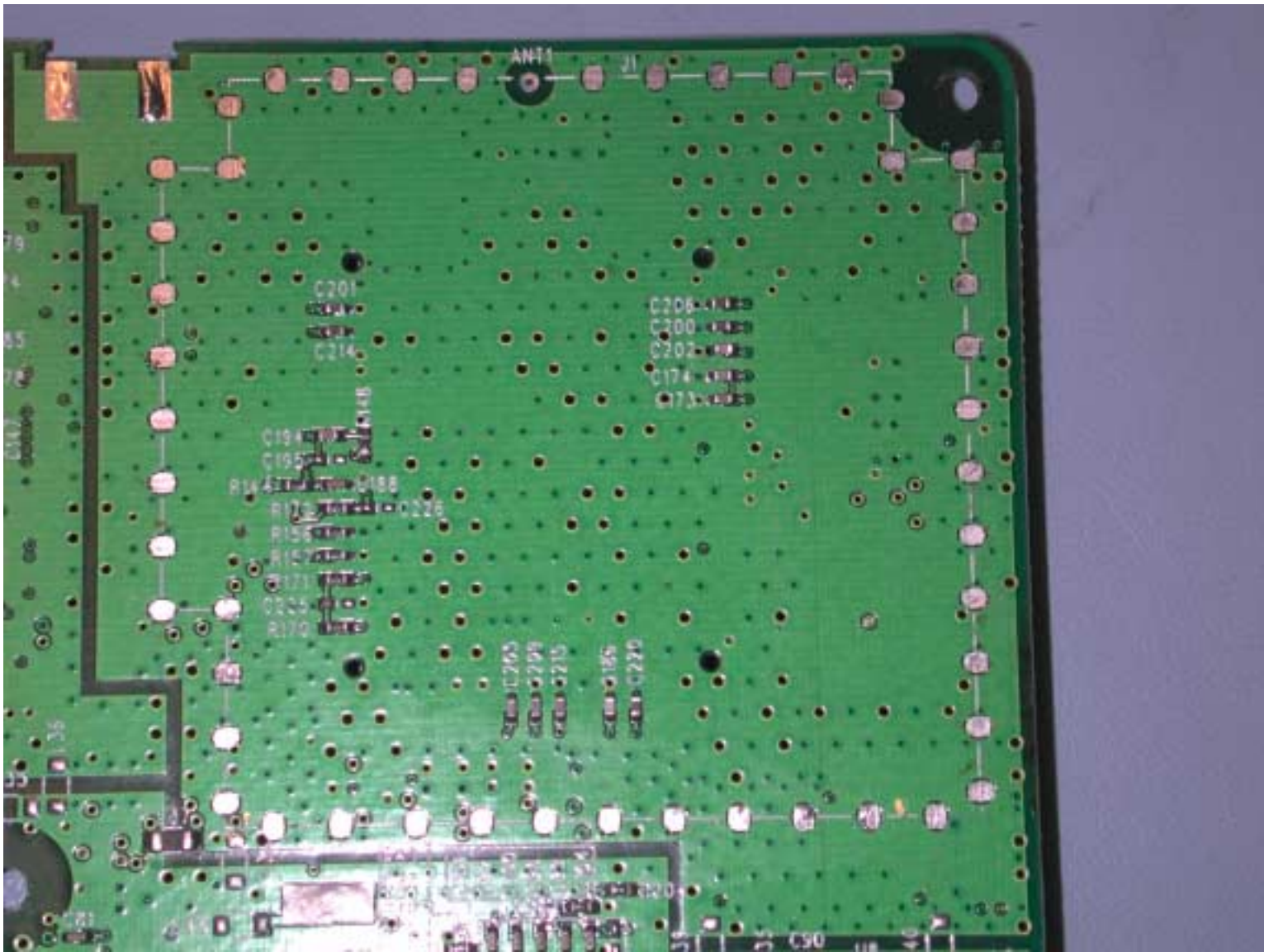
PAB NO ANTENNAS
