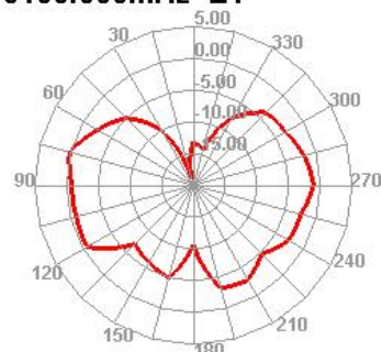
5100.000MHz E1
