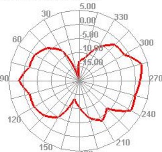
5100.000MHz E2
