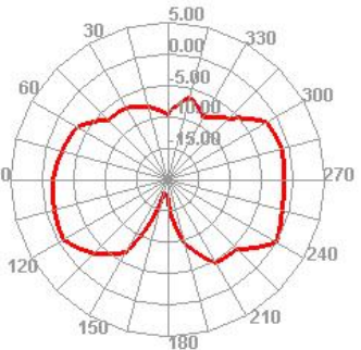
5500.000MHz E2
