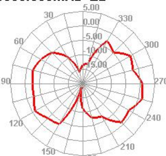
5850.000MHz E2
