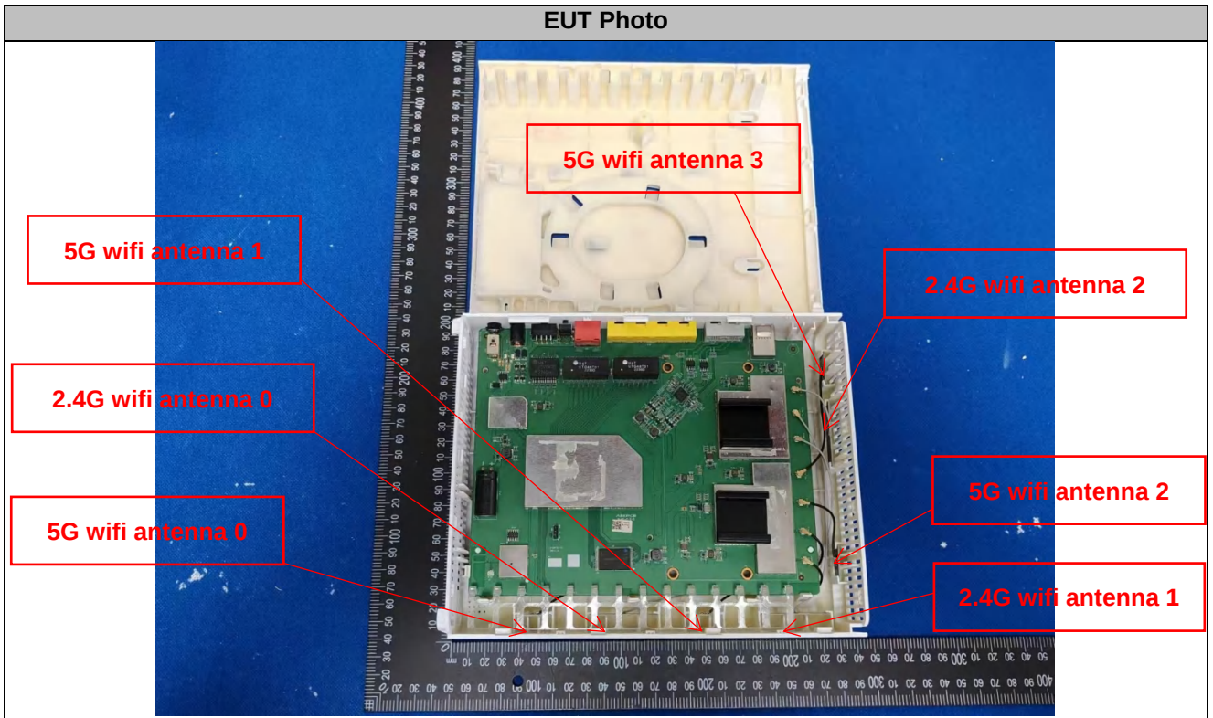
EUT Photo
