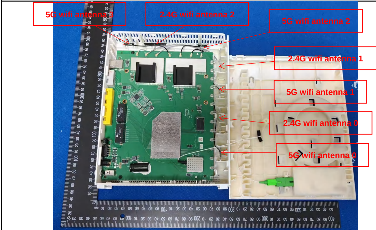
EUT Photo
