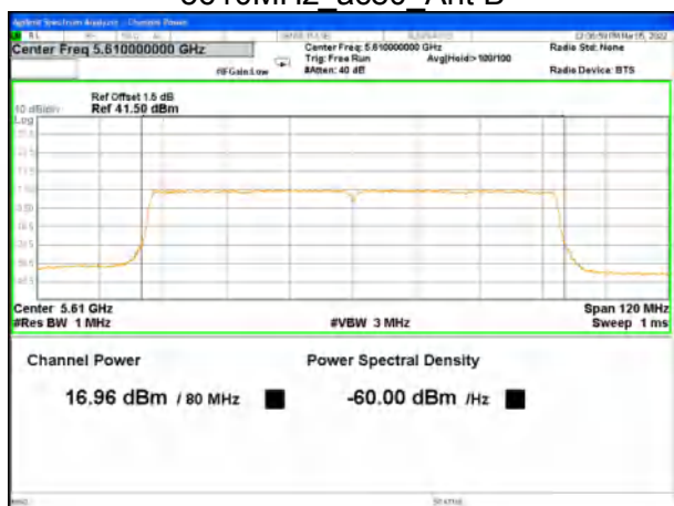
5610MHz_ax80_Ant B
