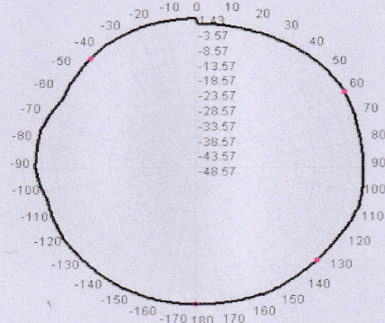
925.0MHz Total(E2-YZ), Max= 1.43dBi
