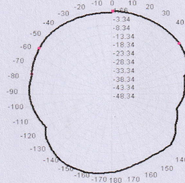
905.0MHz Total(E1-XZ), Max= 0.14dBi
