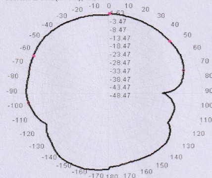
930.0MHz Total(E1-XZ), Max=-0.11dBi
