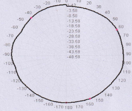
920.0MHz Total(E2-YZ), Max= 1.42dBi
