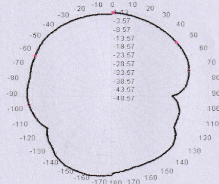
925.0MHz Total(E1-XZ), Max=-0.17dBi
