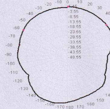
915.0MHz Total(E1-XZ), Max= -0.11dBi
