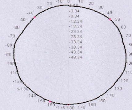
905.0MHz Total(E2-YZ), Max= 1.66dBi
