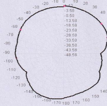
920.0MHz Total(E1-XZ), Max= -0.21dBi
