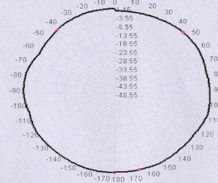
915.0MHz Total(E2-YZ), Max= 1.45dBi
