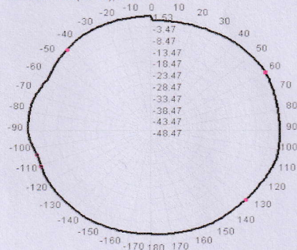
930.0MHz Total(E2-YZ), Max= 1.53dBi
