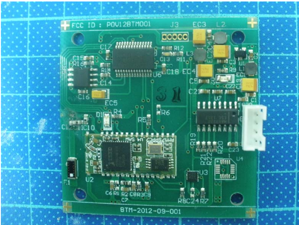
RF module
