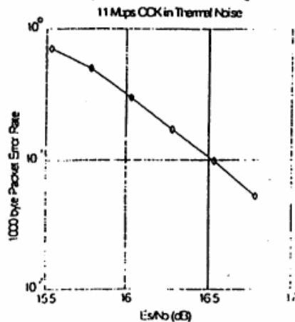
figure.1 1000 byte PER vs. Es/No
