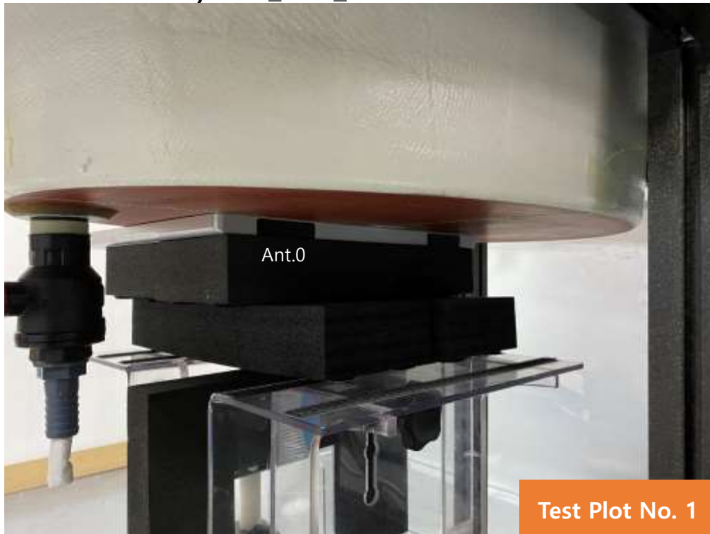
E.1-1) Front_0mm_Ant.0 – 2.4GHz WLAN
