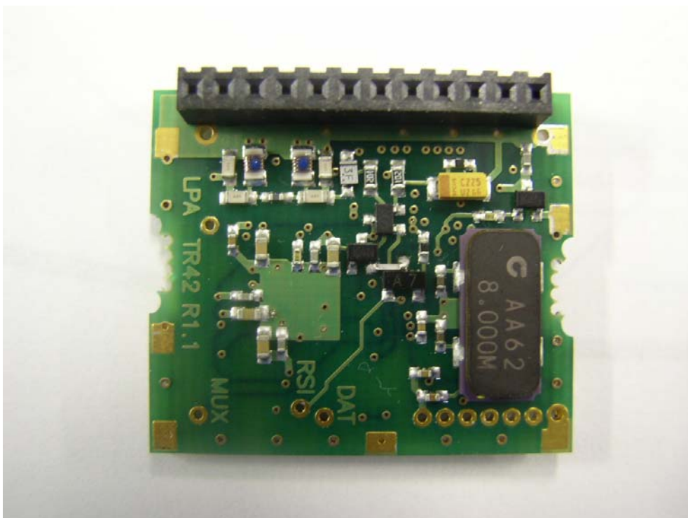
RF Module PCB Bottom View(FCC/IC)
