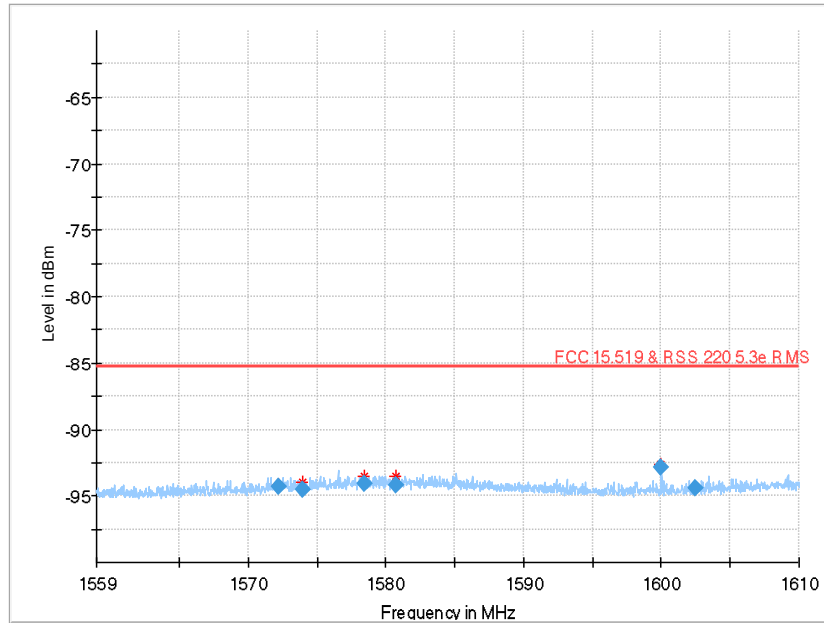
Plot 20: 1559 MHz to 1610 MHz (§15.519 (d), RSS-220 5.3.1(e)), CH 5
