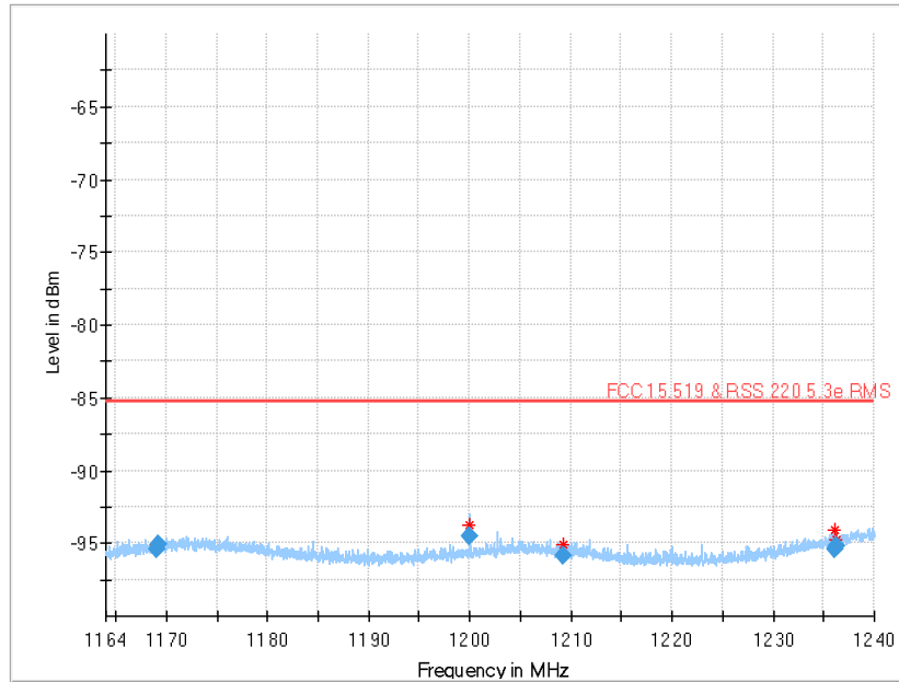
Plot 21: 1164 MHz to 1240 MHz (§15.519 (d), RSS-220 5.3.1(e)), CH 9
