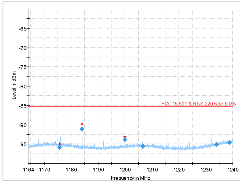
Plot 19: 1164 MHz to 1240 MHz (§15.519 (d), RSS-220 5.3.1(e)), CH 5
