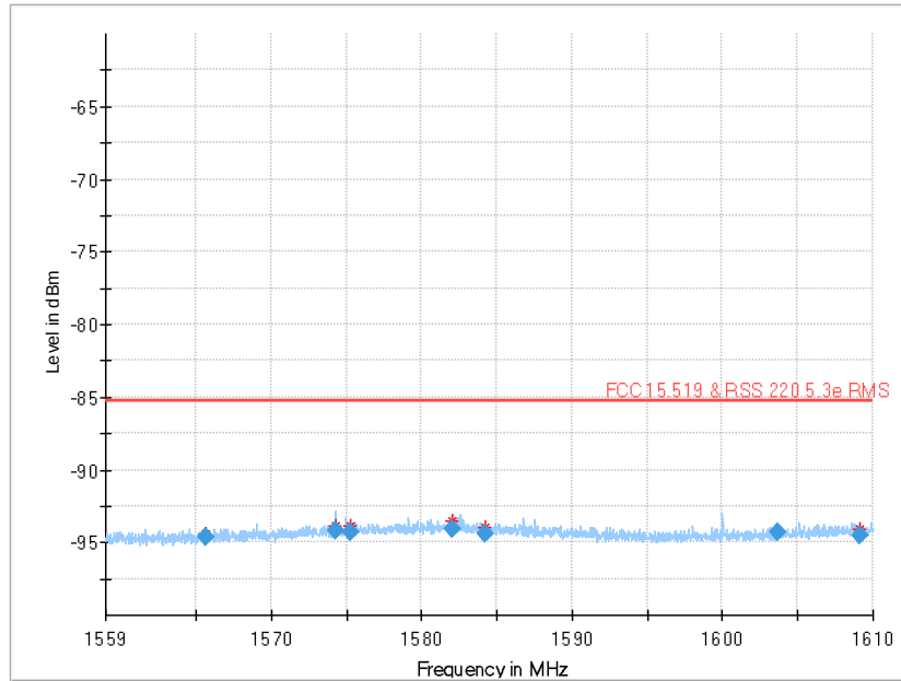
Plot 22: 1559 MHz to 1610 MHz (§15.519 (d), RSS-220 5.3.1(e)), CH 9
