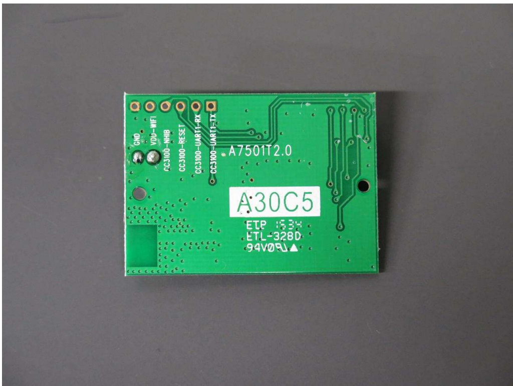
WiFi module
