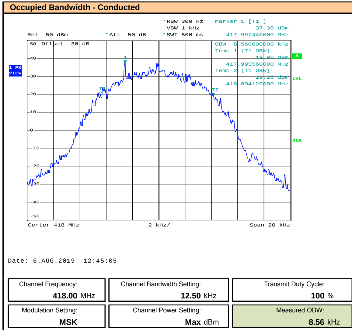
Plot 8.8 – OBW - 12.5kHz BW – MSK – 418MHz , ISED
