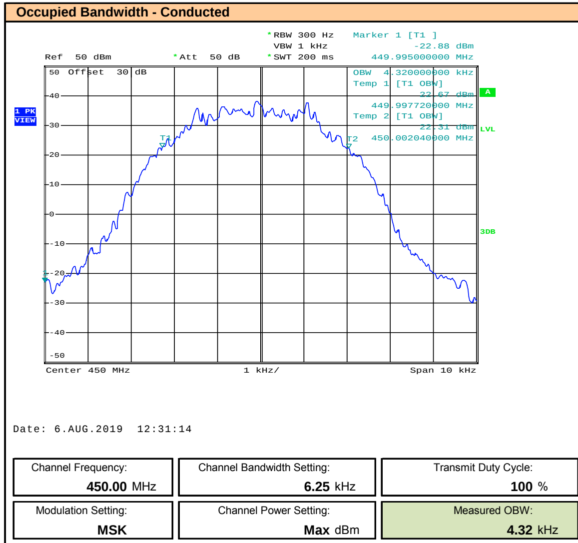
Plot 8.4 – OBW - 6.25kHz BW – MSK - 450MHz
