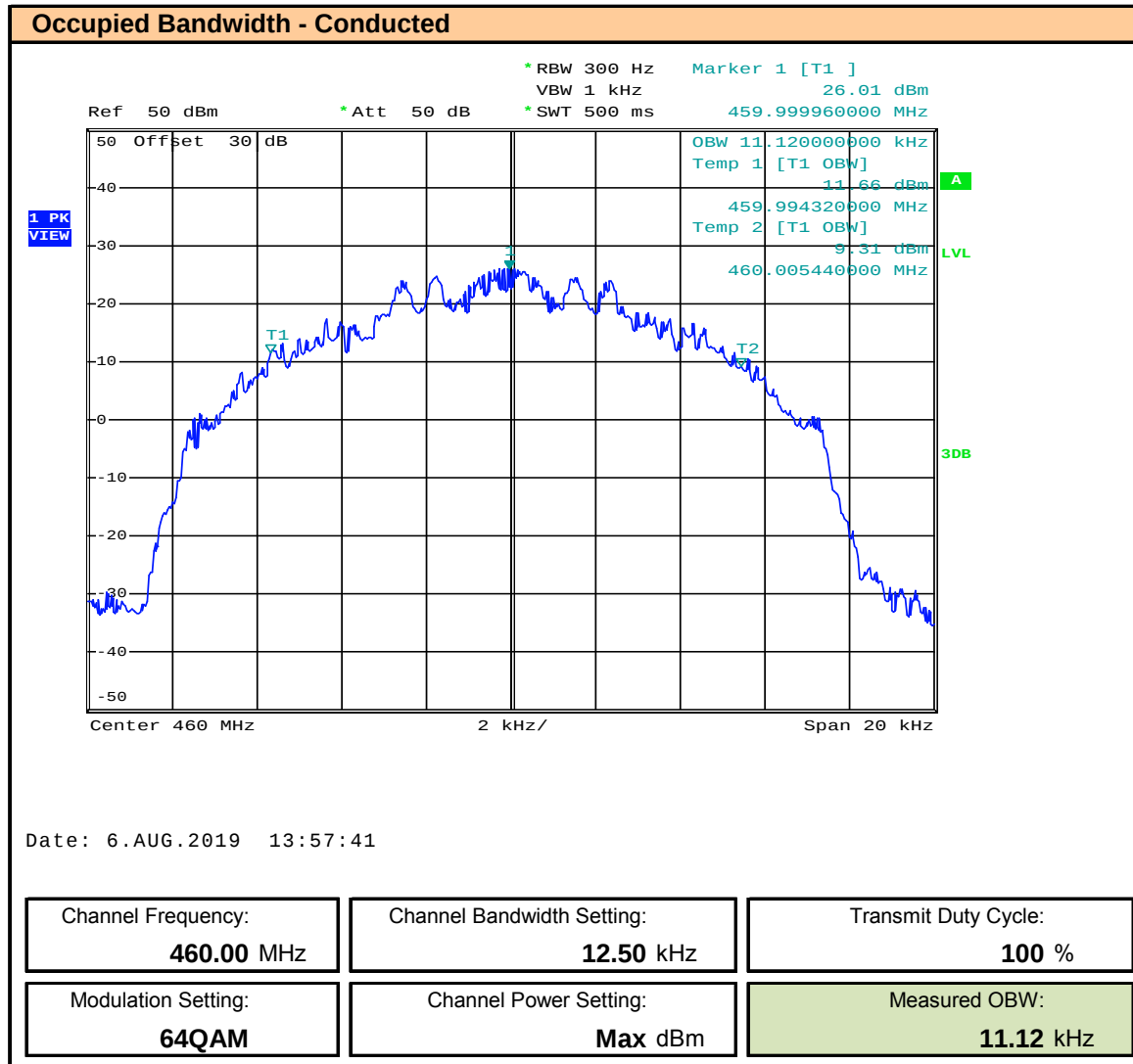
Plot 8.41 – OBW - 12.5kHz BW – 64QAM – 460MHz
