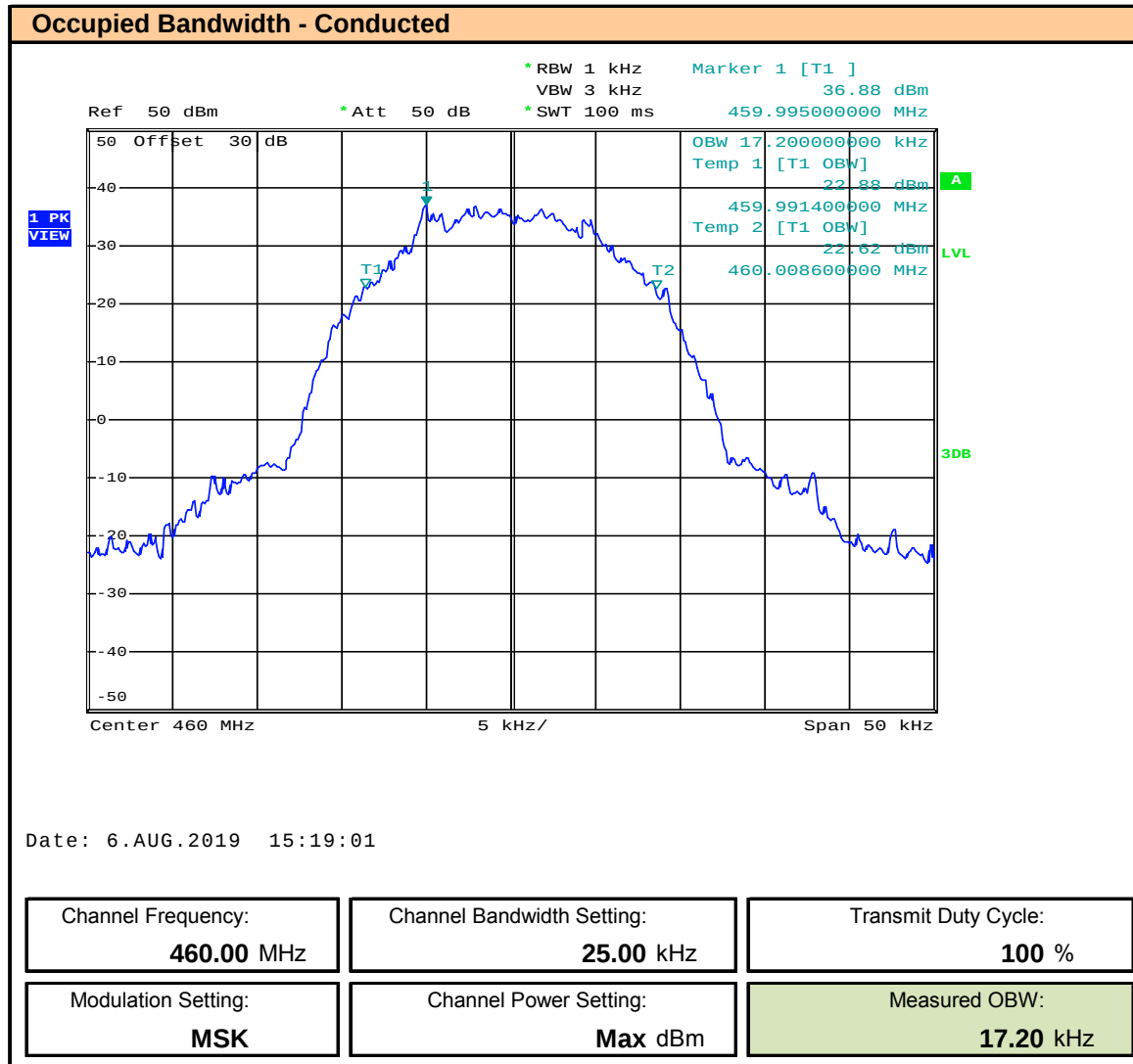
Plot 8.47 – OBW - 25kHz BW – MSK – 460MHz
