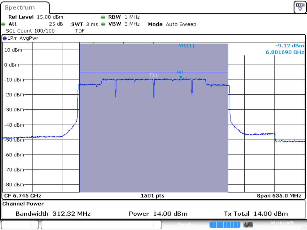
UNII7 MIMO A 802.11be320 ch159 6745MHz
