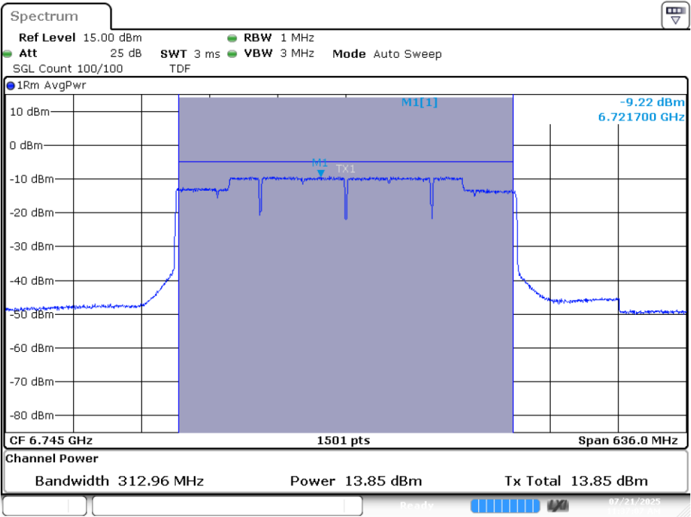
UNII7 MIMO B 802.11be320 ch159 6745MHz
