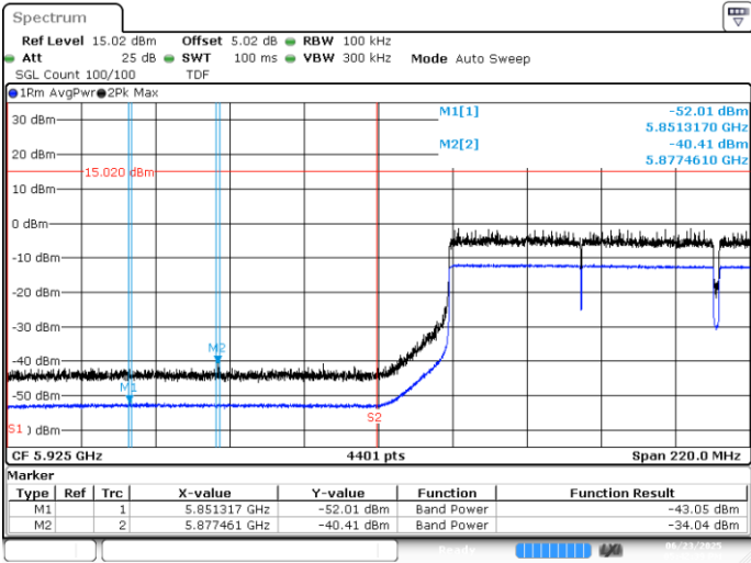
BE-NR-LOW, SISO-A, 802.11be/ax160-MCS0, Ch15
