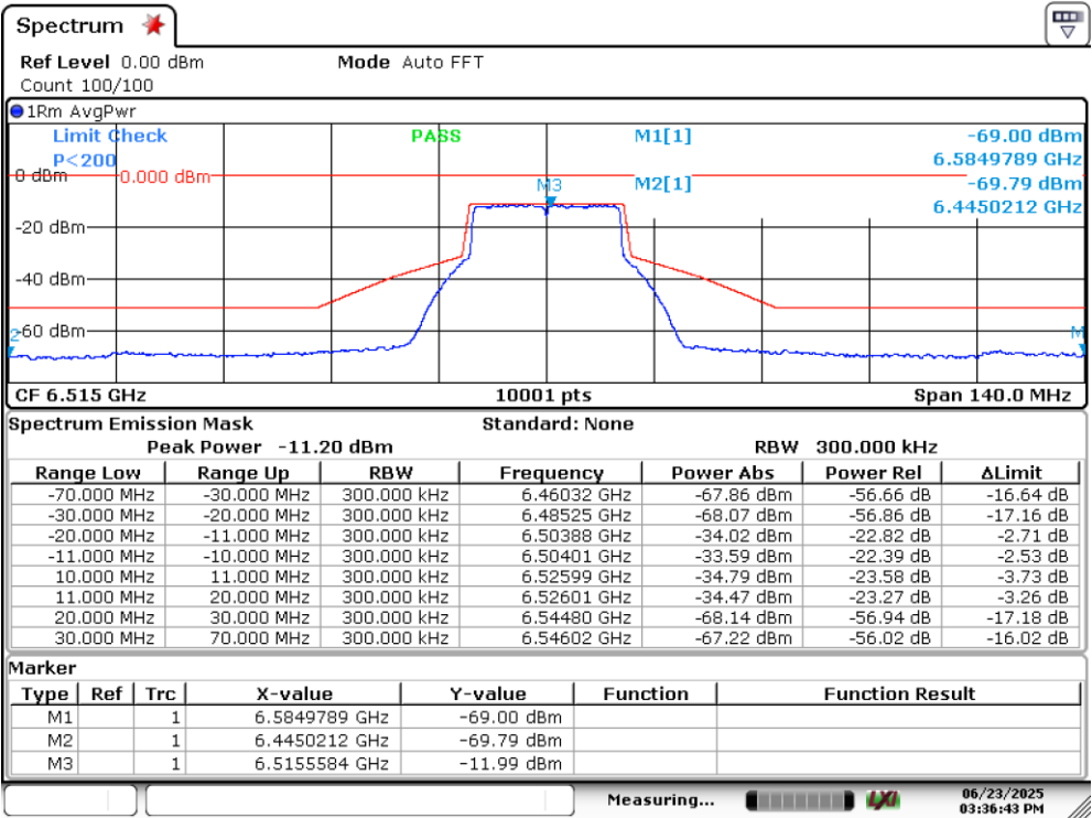
UNI6 SISO B 802.11ax20 ch113 6515MHz
