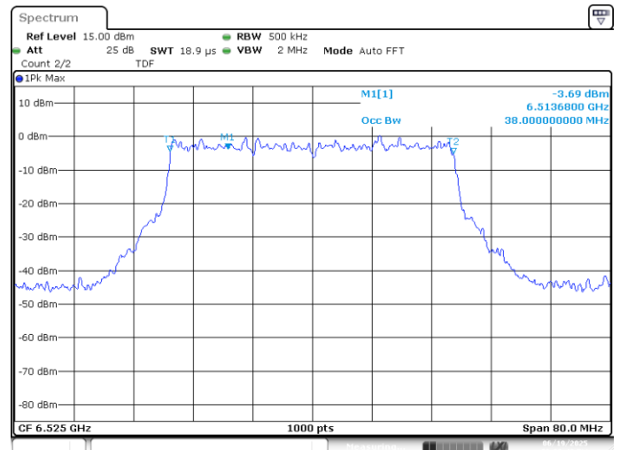
UNII7 SISO B 802.11ax40 ch115 6525MHz 99%
