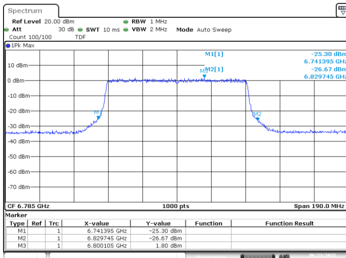
UNII7 MIMO A 802.11ax80 ch167 6785MHz 26dB
