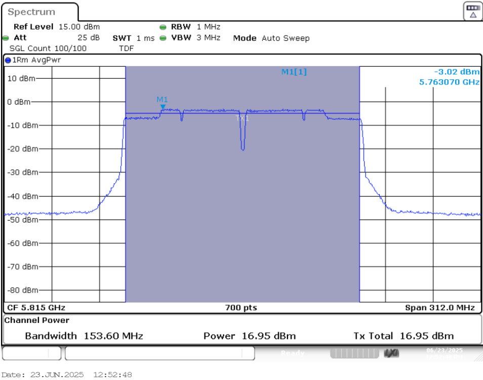
MIMO A-802.11ac160-Ch163-5815MHz-VHT0
