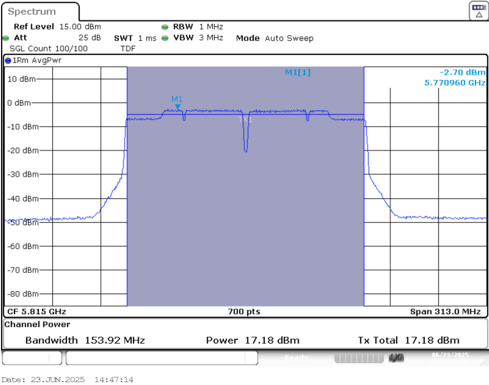
MIMO B-802.11ac160-Ch163-5815MHz-VHT0
