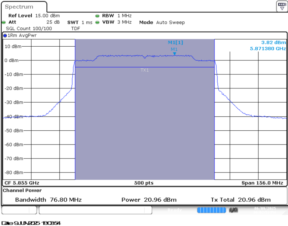
MIMO B-802.11ax/be80-Ch171-5855MHz-MCS0
