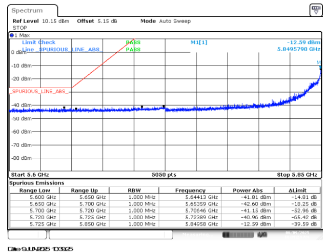
BE-NR-LOW, SISO-A, 802.11ax/be20-HE0, Ch173
