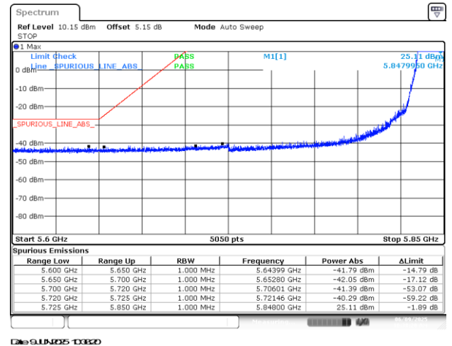
BE-NR-LOW, SISO-A, 802.11ax/be20-HE0, Ch169
