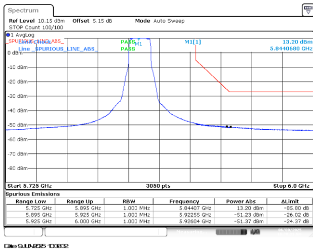
BE-NR-HIGH, SISO-A, 802.11ax/be20-HE0, Ch169
