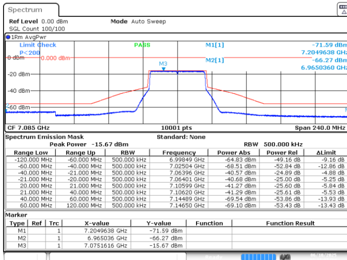
UNII8 MIMO A-802.11ax-40MHz-Ch227-7085MHz-MCS0
