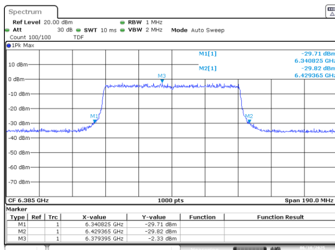
UNII5 MIMO A 802.11ax80 ch87 6385MHz 26dB
