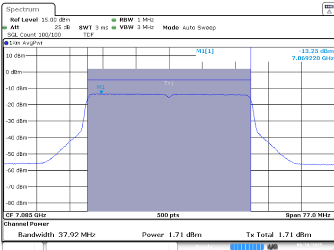
UNII8 MIMO A-802.11ax-40MHz-Ch227-7085MHz-MCS0
