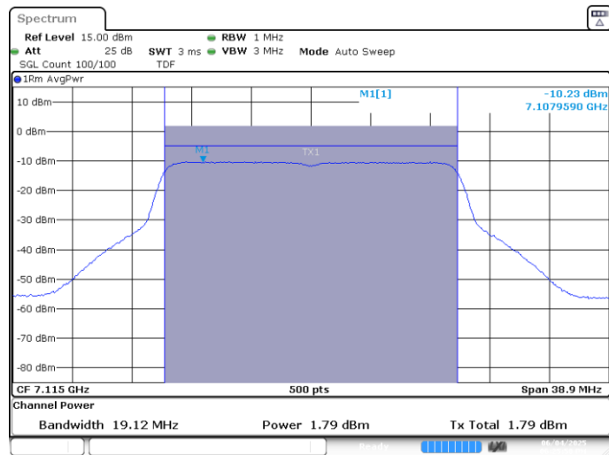
UNII8 SISO A-802.11ax-20MHz-Ch233-7115MHz-MCS0
