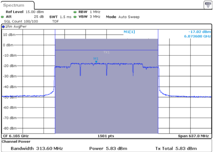
UNII5 MIMO B-802.11be-320MHz-Ch31-6105MHz-MCS0
