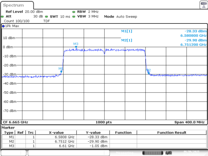
UNII7 MIMO B 802.11ax160 ch143 6665MHz 26dB
