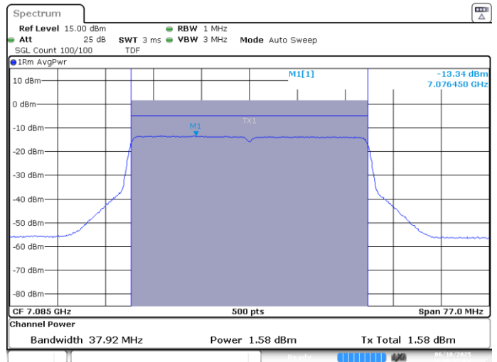
UNII8 MIMO B-802.11ax-40MHz-Ch227-7085MHz-MCS0
