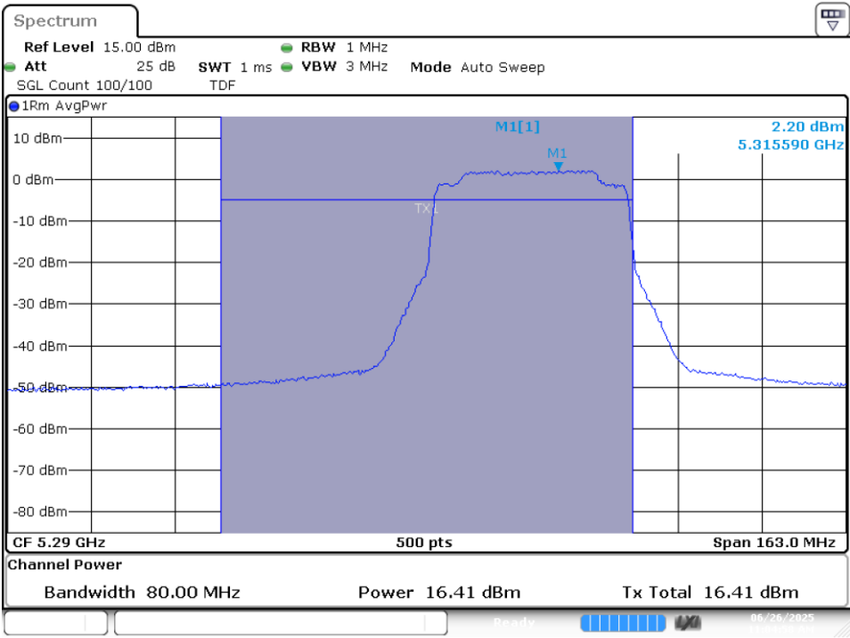
MIMO B-802.11ax/be80-Ch58-5290MHz-MCS0
