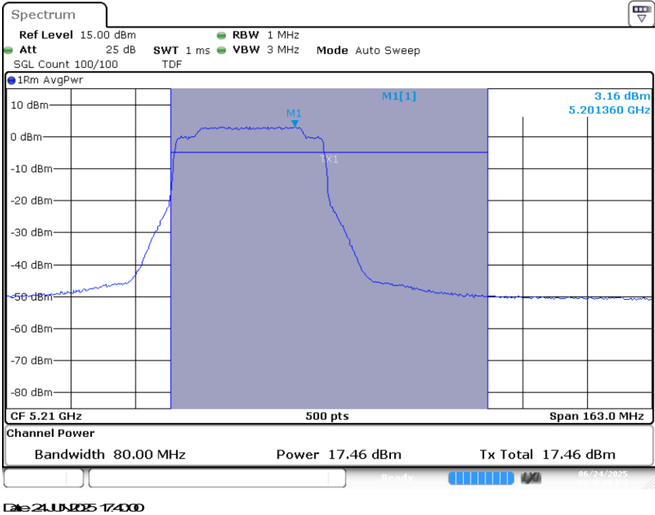
MIMO A-802.11ax/be80-Ch42-5210MHz-MCS0
