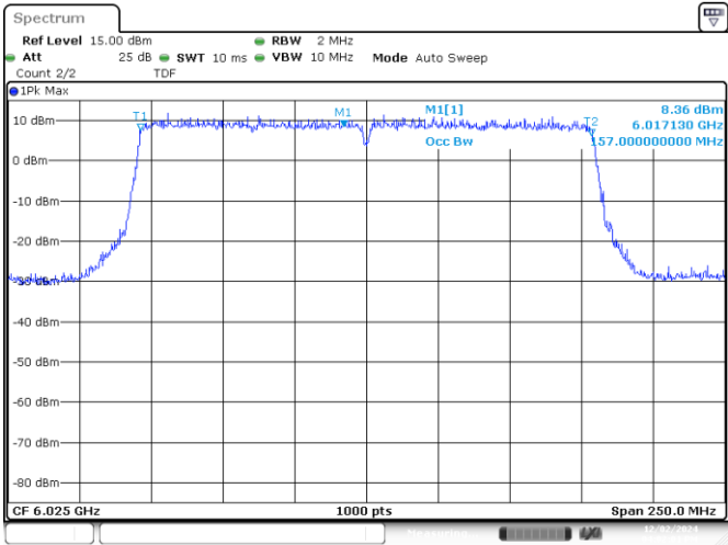
UNII5 MIMO A 802.11ax/be160 ch15 6025MHz 99%
