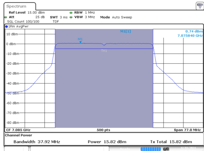
SISO B-802.11ax/be-40MHz-Ch227-7085MHz-MCS0
