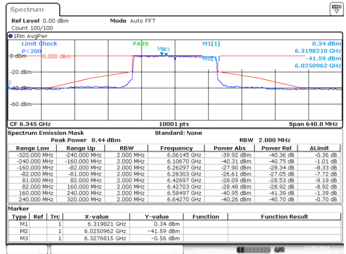
MIMO B-802.11ax/be-160MHz-Ch79-6345MHz-MCS0
