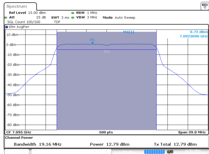
SISO B-802.11ax/be-20MHz-Ch229-7095MHz-MCS0
