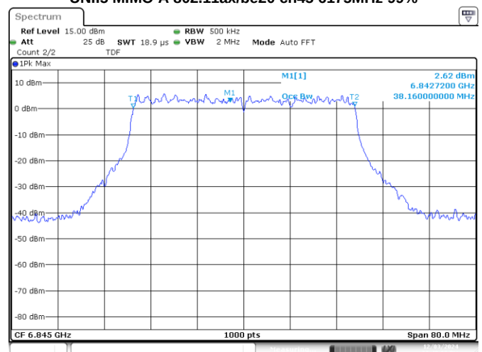
UNII7 SISO B 802.11ax/be40 ch179 6845MHz 99%
