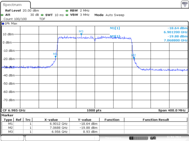
UNII8 MIMO A 802.11ax/be160 ch207 6985MHz 26dB
