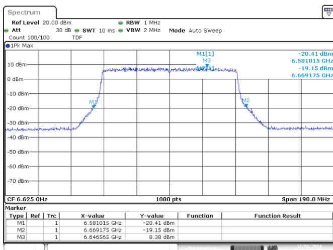
UNII7 MIMO A 802.11ax/be80 ch135 6625MHz 26dB
