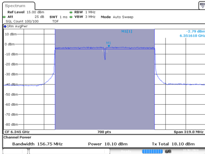
MIMO A-802.11ax/be-160MHz-Ch79-6345MHz-MCS0
