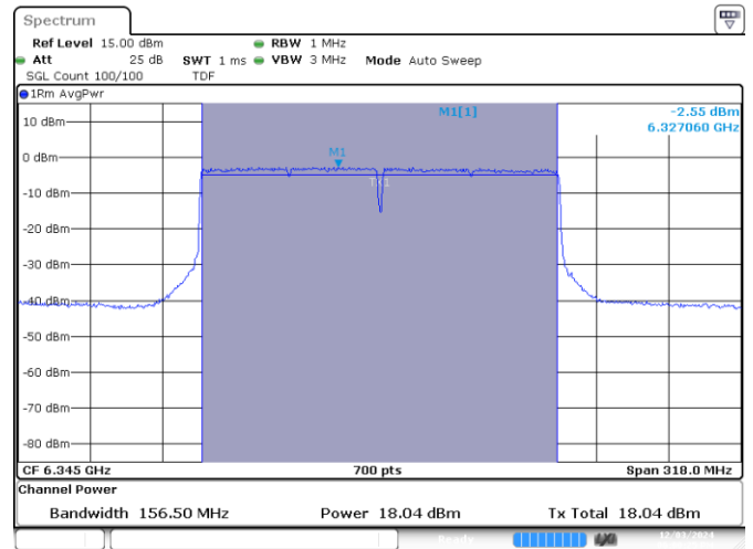
MIMO B-802.11ax/be-160MHz-Ch79-6345MHz-MCS0
