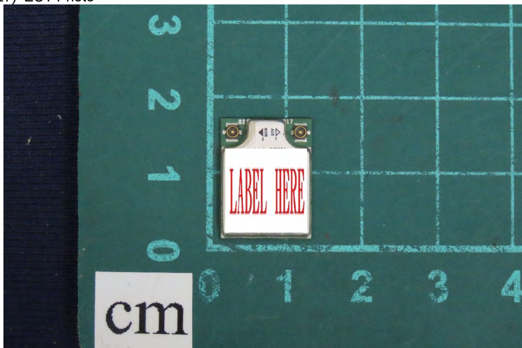
(17) EUT Photo
