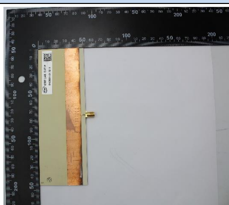
Antenna 5 GHz
