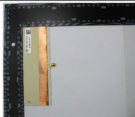
Antenna 5 GHz
