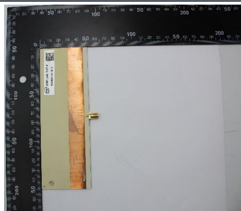
Antenna 5 GHz
