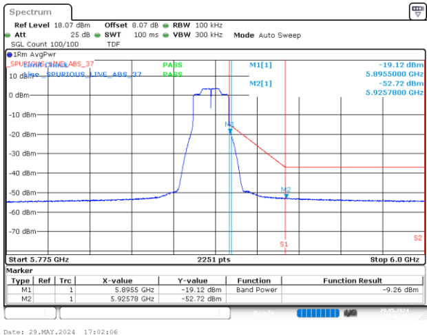
BE-NR-HIGH, MIMO-A, 802.11ax/be20-MCS0, Ch177
