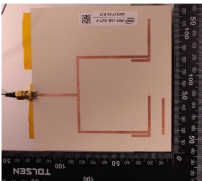
Antenna 2.4 GHz
