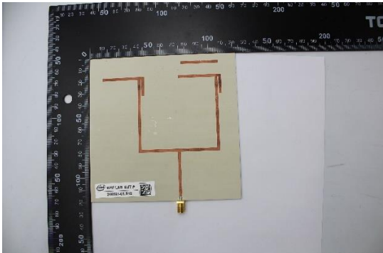
Antenna 2.4 GHz
