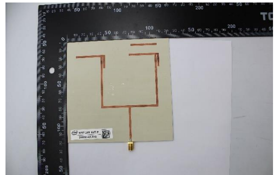
Antenna 2.4 GHz
