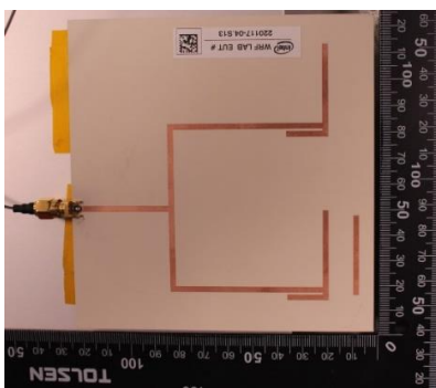
Antenna 2.4 GHz
