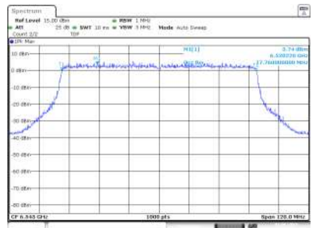
SISO A 802.11ax/be80 ch119 99%
