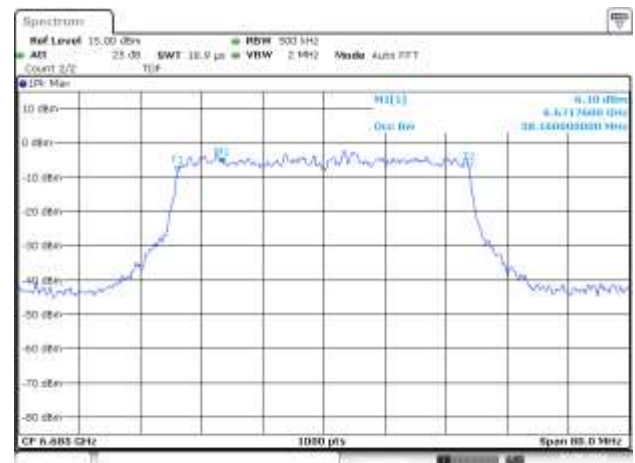
MIMO A 802.11ax/be40 ch147 99%
