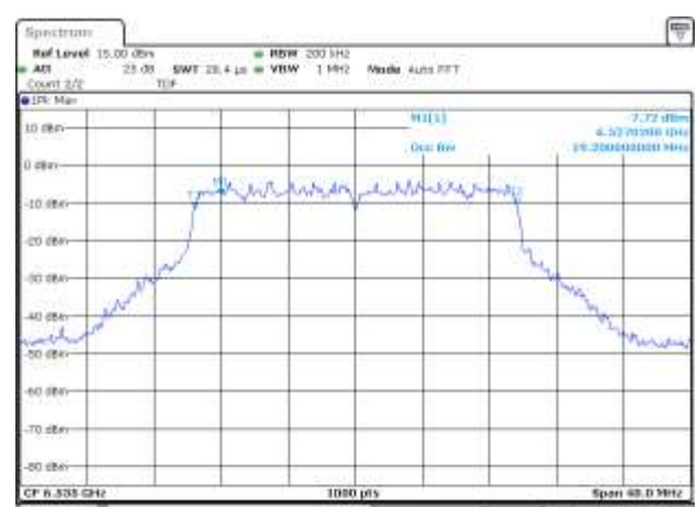
SISO B 802.11ax/be20 ch117 99%
