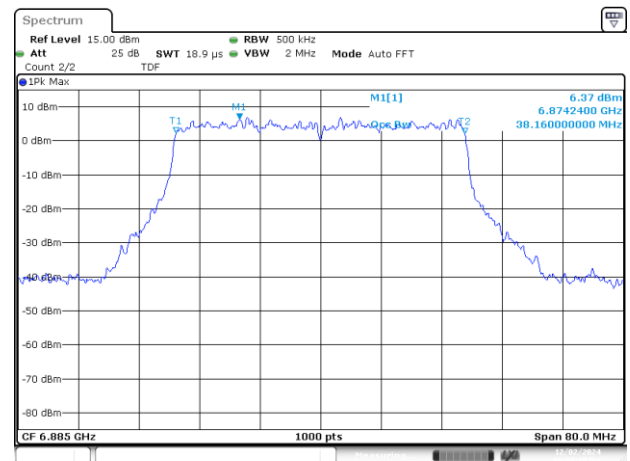
UNII8 SISO B 802.11ax/be40 ch187 6885MHz 99%
