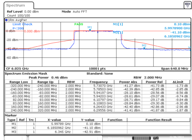
MIMO B-802.11ax/be-160MHz-Ch15-6025MHz-MCS0
