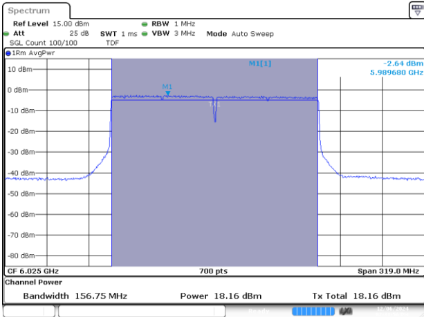
MIMO B-802.11ax/be-160MHz-Ch15-6025MHz-MCS0
