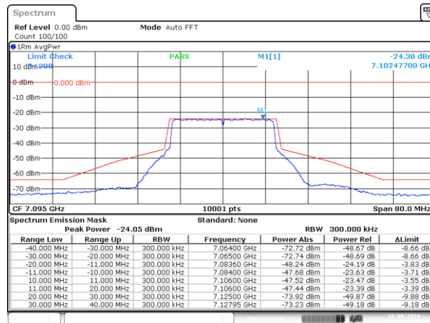
SISO A-802.11ax/be-20MHz-Ch229-7095MHz-MCS0
