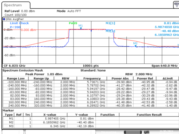
MIMO A-802.11ax/be-160MHz-Ch15-6025MHz-MCS0
