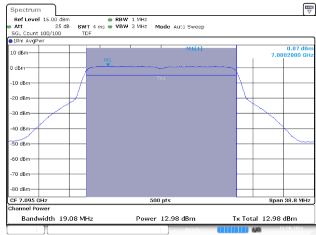
SISO A-802.11ax/be-20MHz-Ch229-7095MHz-MCS0
