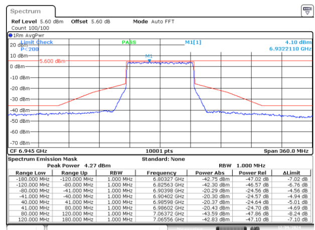
MIMO B-802.11ax/be-80MHz-Ch199-6945MHz-MCS0
