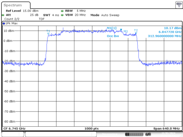
UNII7 SISO B 802.11be320 ch159 6745MHz 99%
