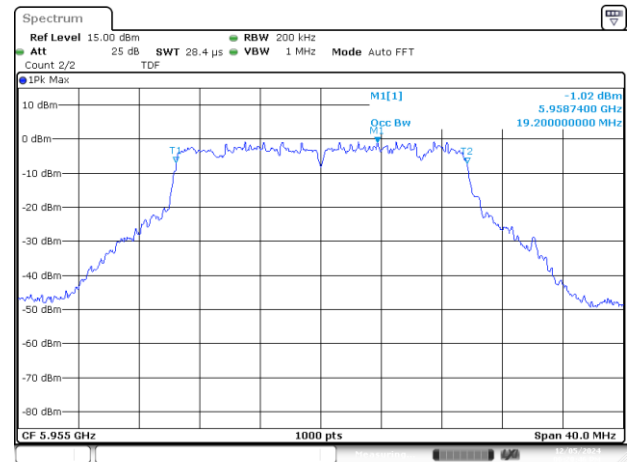
UNII5 MIMO A 802.11ax/be20 ch1 5955MHz 99%
