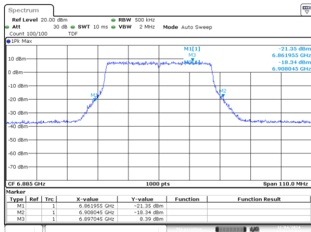
UNII8 SISO A 802.11ax/be40 ch187 6885MHz 26dB
