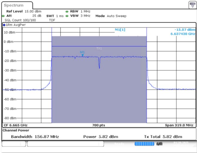
MIMO B-802.11ax/be-160MHz-Ch143-6665MHz-MCS0
