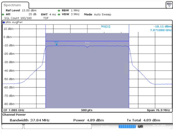
SISO A-802.11ax/be-40MHz-Ch227-7085MHz-MCS0
