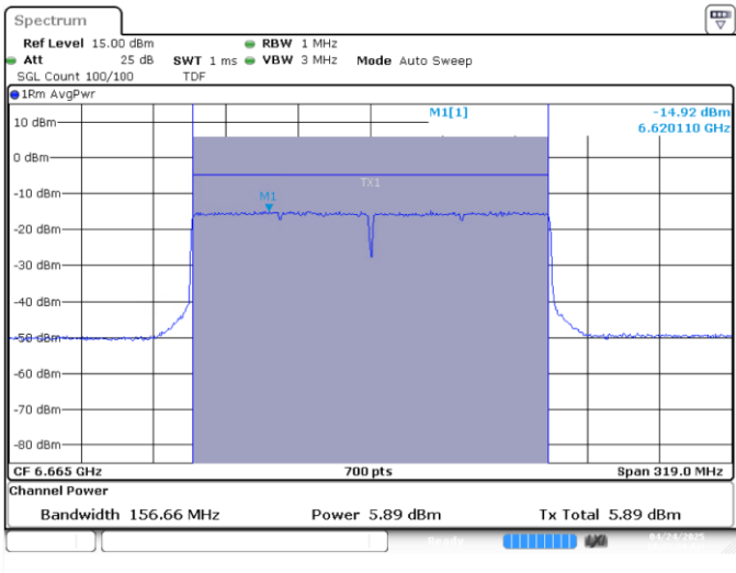
MIMO A-802.11ax/be-160MHz-Ch143-6665MHz-MCS0
