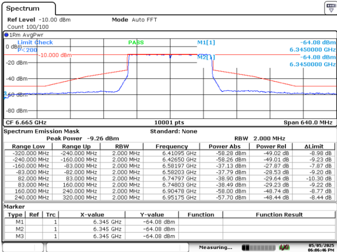
MIMO A-802.11ax/be-160MHz-Ch143-6665MHz-MCS0
