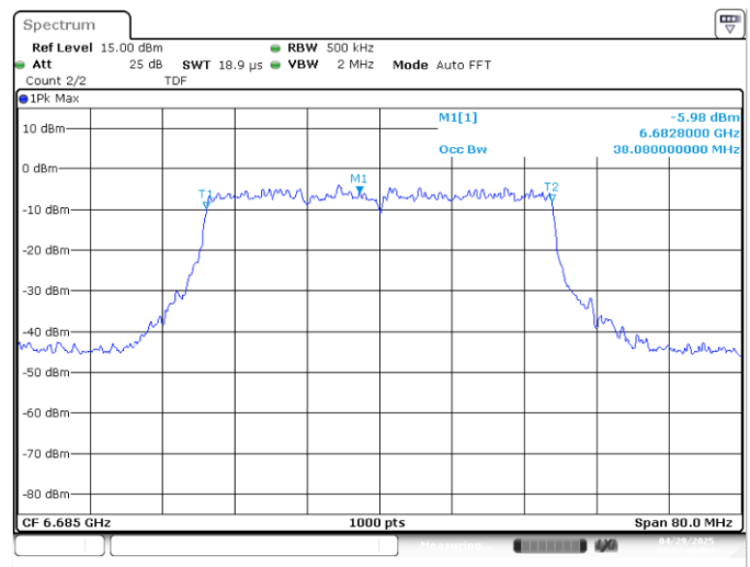
UNII5 SISO B 802.11ax/be40 ch147 6685MHz 99%
