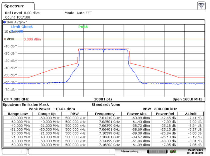
SISO A-802.11ax/be-40MHz-Ch227-7085MHz-MCS0
