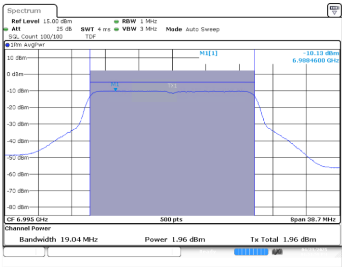
SISO A-802.11ax/be-20MHz-Ch209-6995MHz-MCS0
