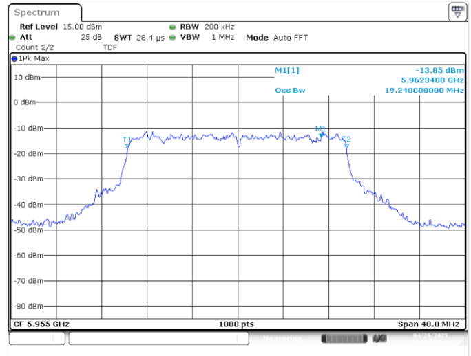
UNII5 MIMO B 802.11ax/be20 ch1 5955MHz 99%
