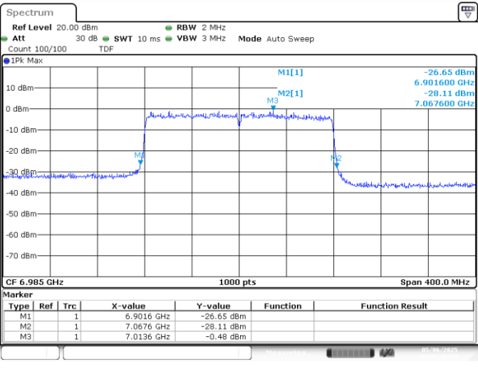
UNII8 MIMO B 802.11ax/be160 ch207 6985MHz 26dB
