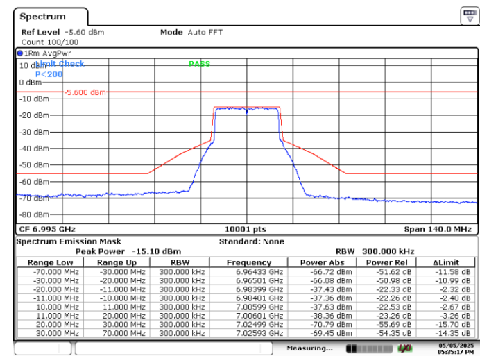
SISO A-802.11ax/be-20MHz-Ch209-6995MHz-MCS0
