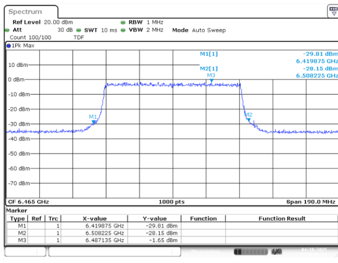
UNII6 MIMO B 802.11ax/be80 ch103 6465MHz 26dB
