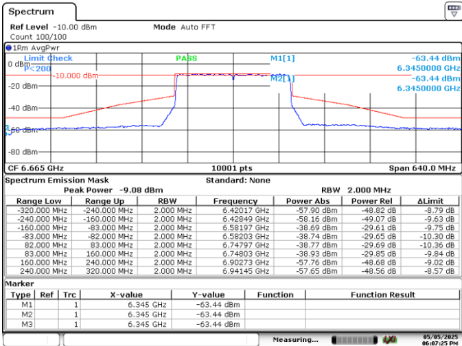
MIMO B-802.11ax/be-160MHz-Ch143-6665MHz-MCS0
