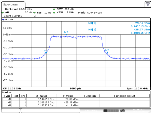
UNII5 MIMO B 802.11ax/be40 ch43 6165MHz 26dB
