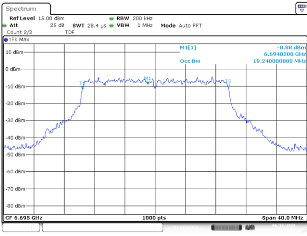
UNII7 SISO A 802.11ax/be20 ch149 6695MHz 99%
