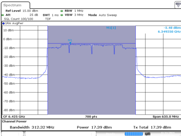
MIMO B-802.11be-320MHz-Ch95-6425MHz-MCS0
