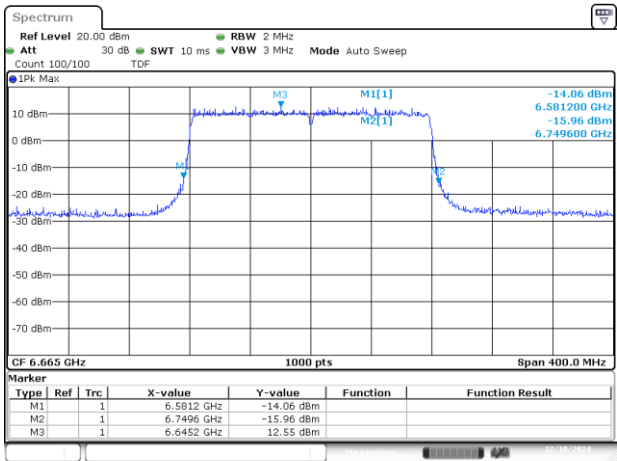
UNII7 SISO A 802.11ax/be160 ch143 6665MHz 26dB
