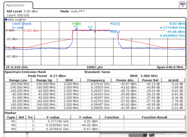
MIMO B-802.11ax/be-160MHz-Ch79-6345MHz-MCS0
