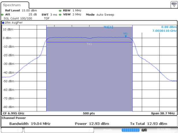
SISO B-802.11ax/be-20MHz-Ch209-6995MHz-MCS0
