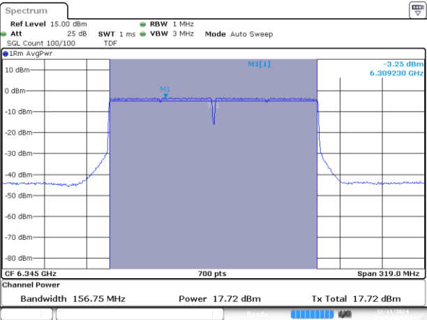
MIMO A-802.11ax/be-160MHz-Ch79-6345MHz-MCS0
