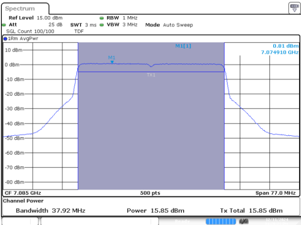
SISO B-802.11ax/be-40MHz-Ch227-7085MHz-MCS0
