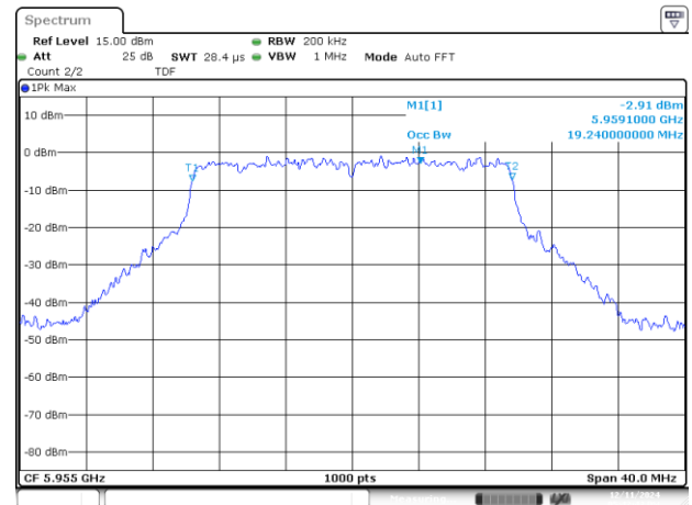
UNII5 MIMO B 802.11ax/be20 ch1 5955MHz 99%
