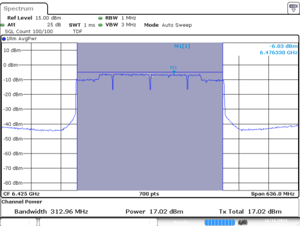
MIMO A-802.11be-320MHz-Ch95-6425MHz-MCS0
