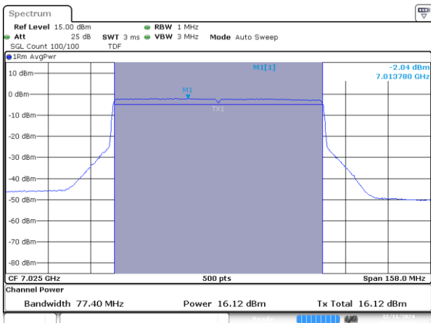
MIMO B-802.11ax/be-80MHz-Ch219-7025MHz-MCS0
