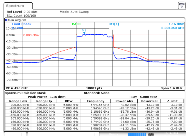
MIMO B-802.11be-320MHz-Ch95-6425MHz-MCS0
