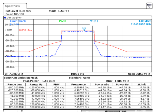
MIMO B-802.11ax/be-80MHz-Ch215-7025MHz-MCS0
