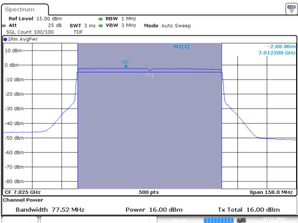
MIMO A-802.11ax/be-80MHz-Ch215-7025MHz-MCS0
