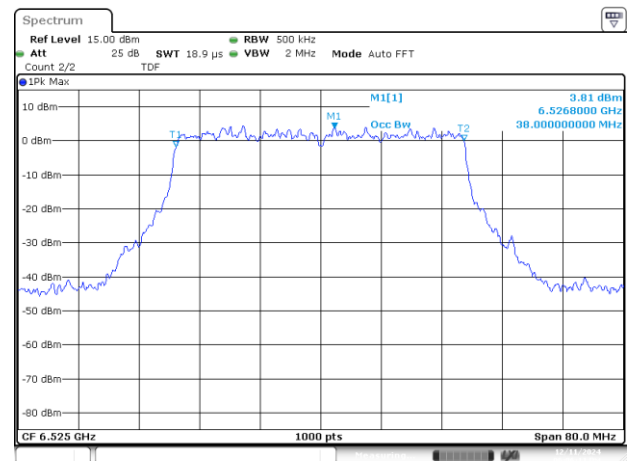
UNII7 MIMO B 802.11ax/be40 ch115 6525MHz 99%
