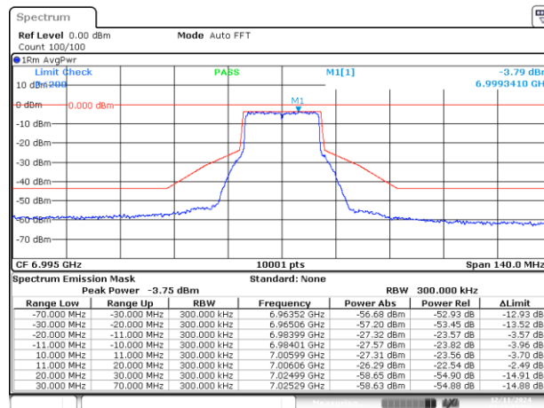
SISO B-802.11ax/be-20MHz-Ch209-6995MHz-MCS0
