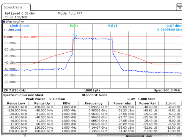
MIMO A-802.11ax/be-80MHz-Ch215-7025MHz-MCS0
