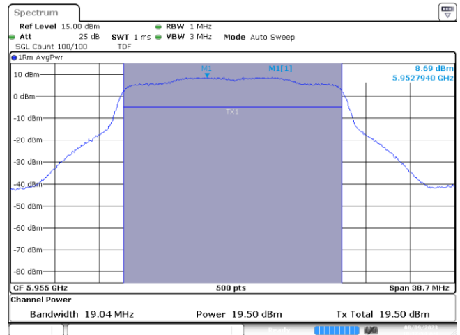
MIMO B-802.11ax/be-20MHz-Ch1-5955MHz-MCS0
