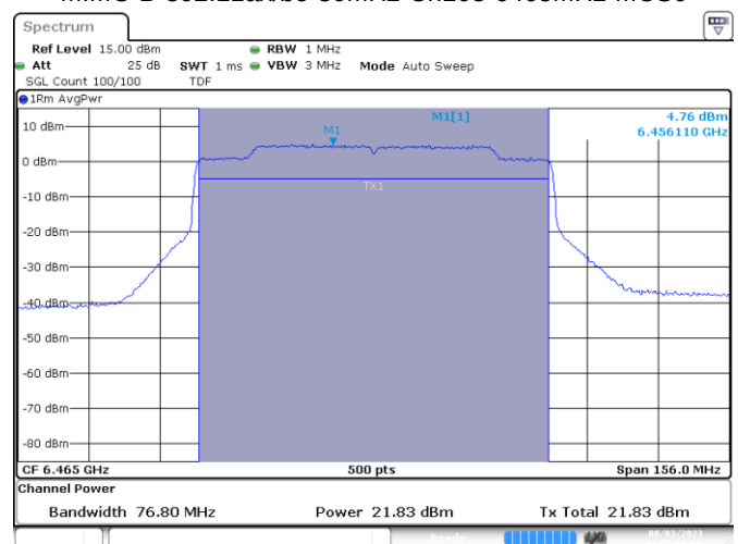
MIMO B-802.11ax/be-80MHz-Ch103-6465MHz-MCS0
