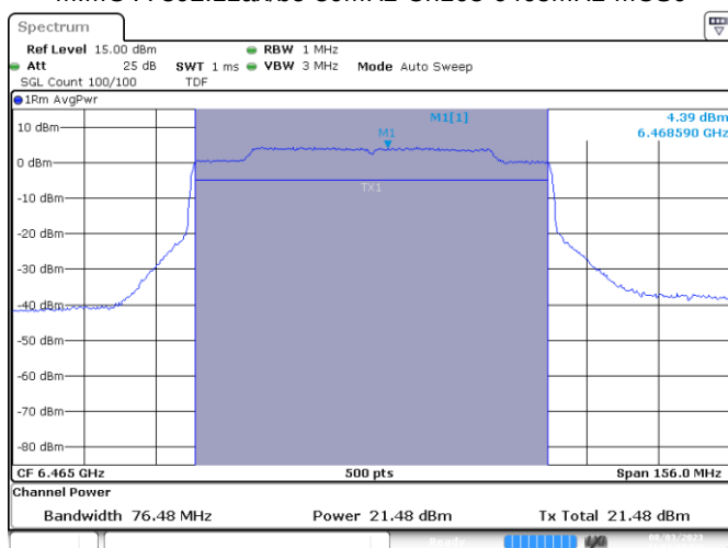
MIMO A-802.11ax/be-80MHz-Ch103-6465MHz-MCS0
