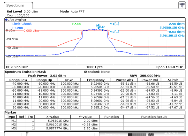
MIMO B-802.11ax/be-20MHz-Ch1-5955MHz-MCS0
