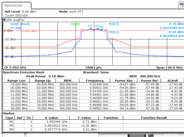
MIMO A-802.11ax/be-20MHz-Ch1-5955MHz-MCS0
