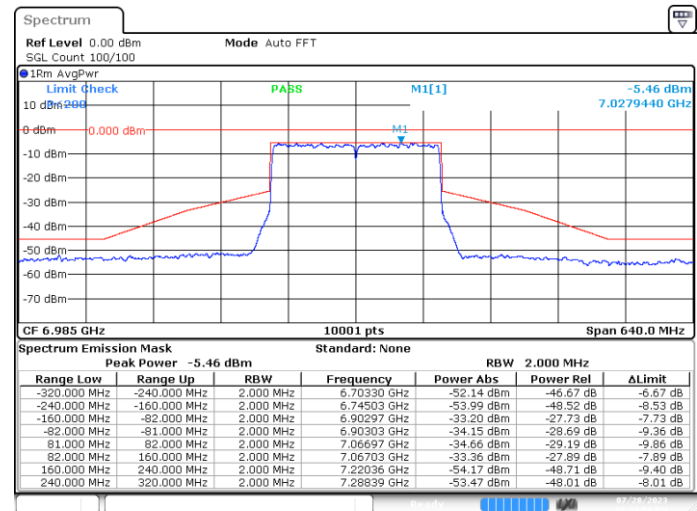
MIMO B-802.11ax/be-160MHz-Ch207-6985MHz-MCS0
