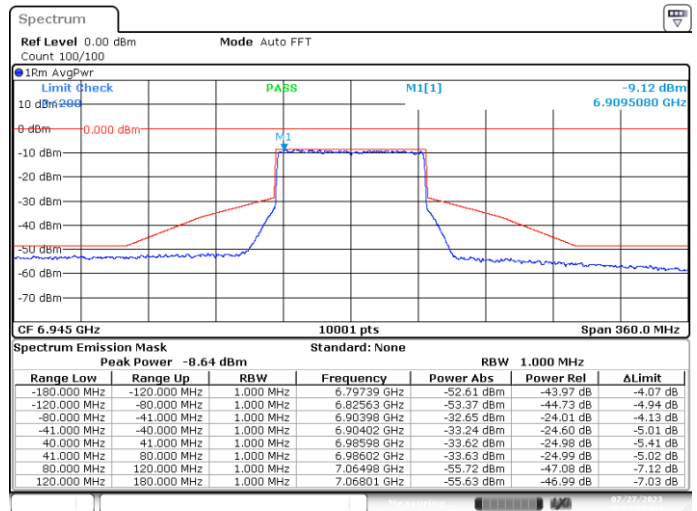
MIMO B-802.11ax/be-80MHz-Ch199-6945MHz-MCS0
