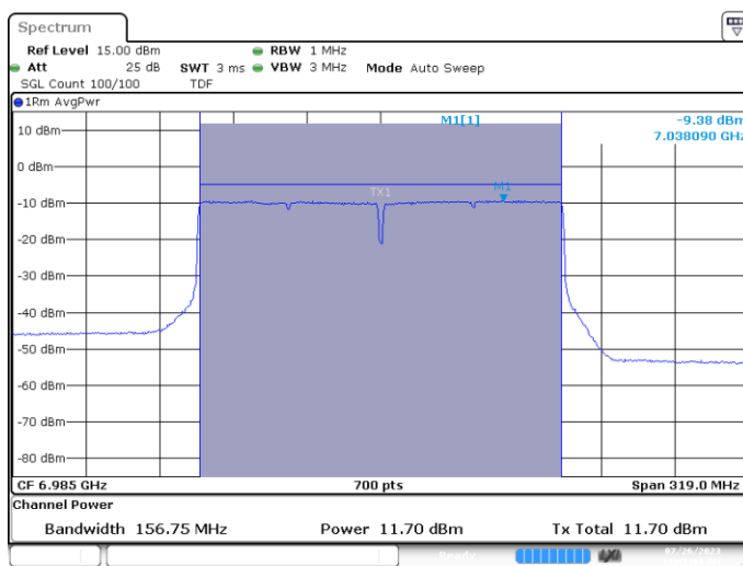
MIMO A-802.11ax/be-160MHz-Ch207-6985MHz-MCS0
