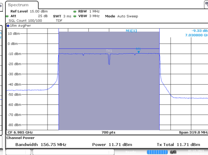
MIMO B-802.11ax/be-160MHz-Ch207-6985MHz-MCS0
