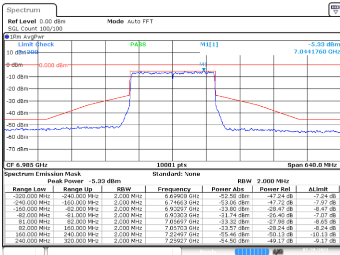
MIMO A-802.11ax/be-160MHz-Ch207-6985MHz-MCS0
