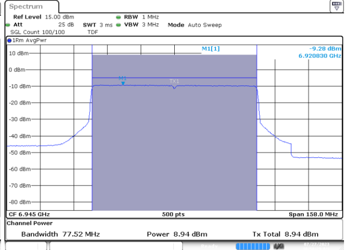
MIMO B-802.11ax/be-80MHz-Ch199-6945MHz-MCS0
