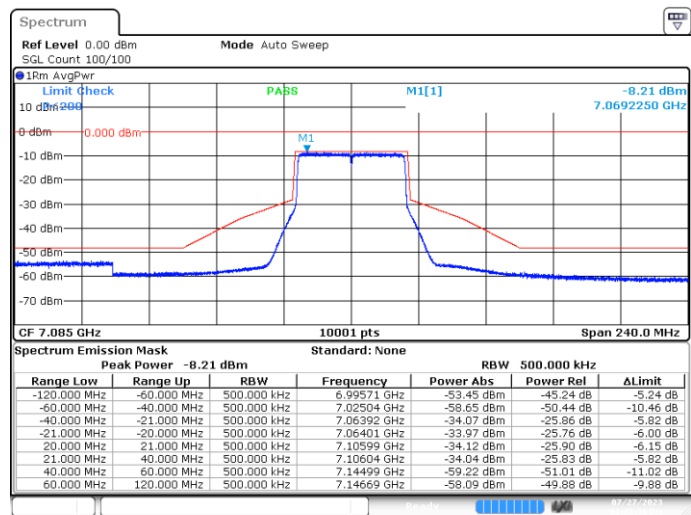
SISO B-802.11ax/be-40MHz-Ch227-7085MHz-MCS0
