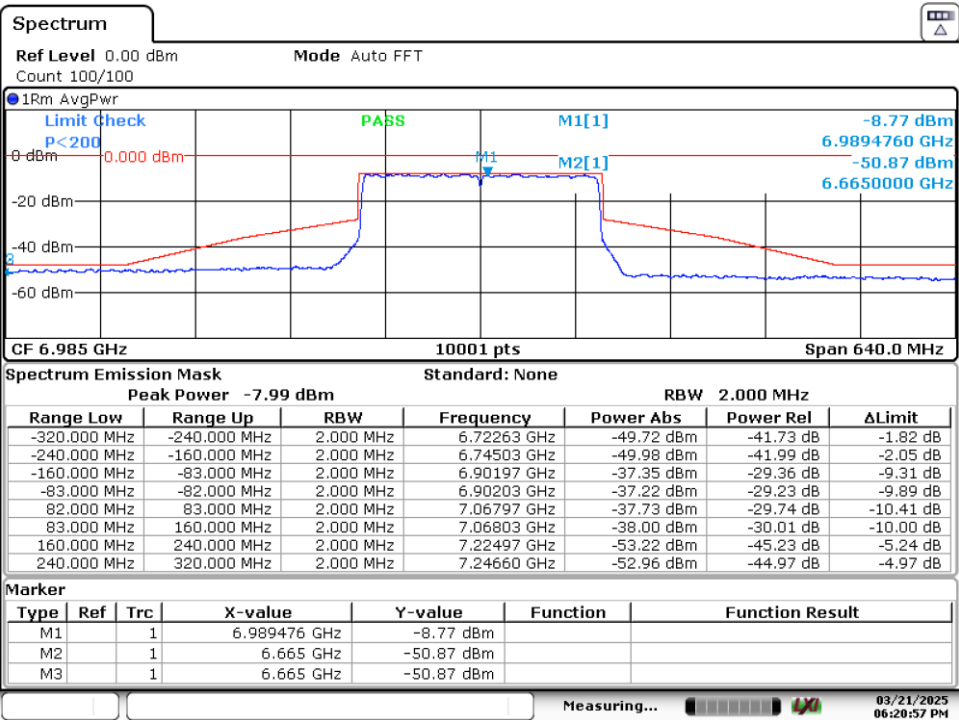
SISO A-802.11ax/be-160MHz-Ch207-6985MHz-MCS0
