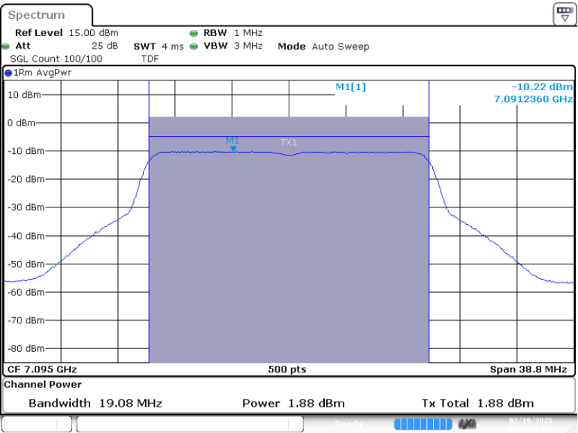
SISO A-802.11ax/be-20MHz-Ch229-7095MHz-MCS0
