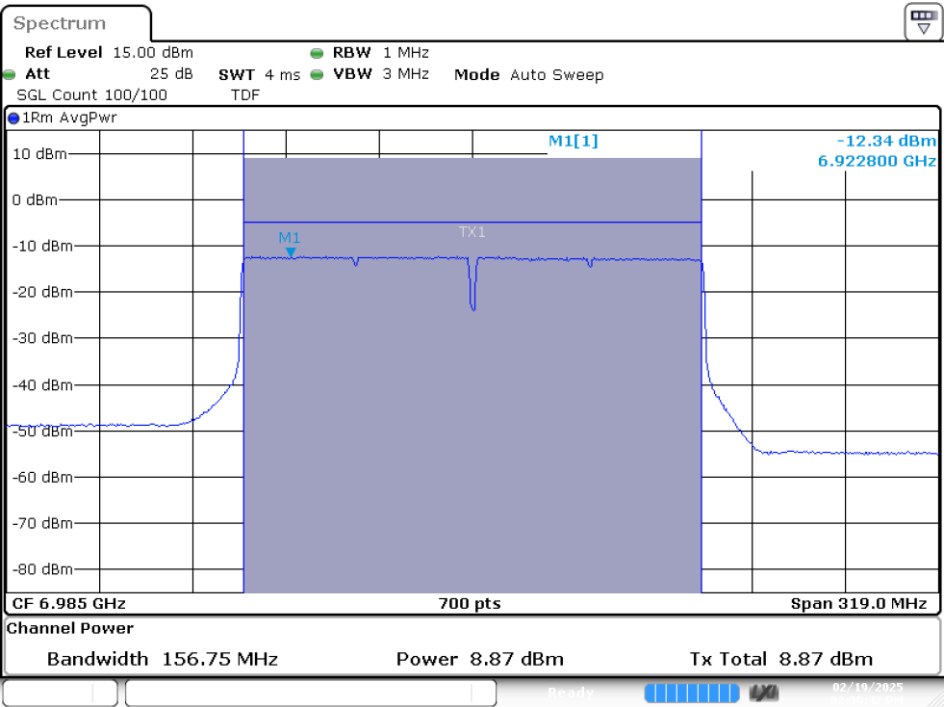
SISO A-802.11ax/be-160MHz-Ch207-6985MHz-MCS0
