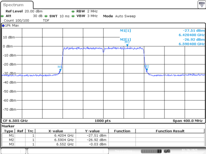
UNII6 MIMO A 802.11ax/be160 ch111 6505MHz 26dB
