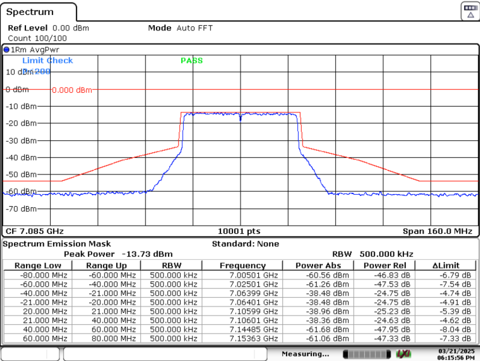
SISO A-802.11ax/be-40MHz-Ch227-7085MHz-MCS0
