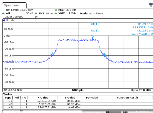
UNII-5 SISO B 802.11ax/be20 ch1 5955MHz 26dB
