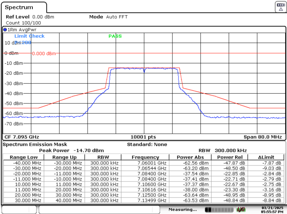
SISO A-802.11ax/be-20MHz-Ch229-7095MHz-MCS0
