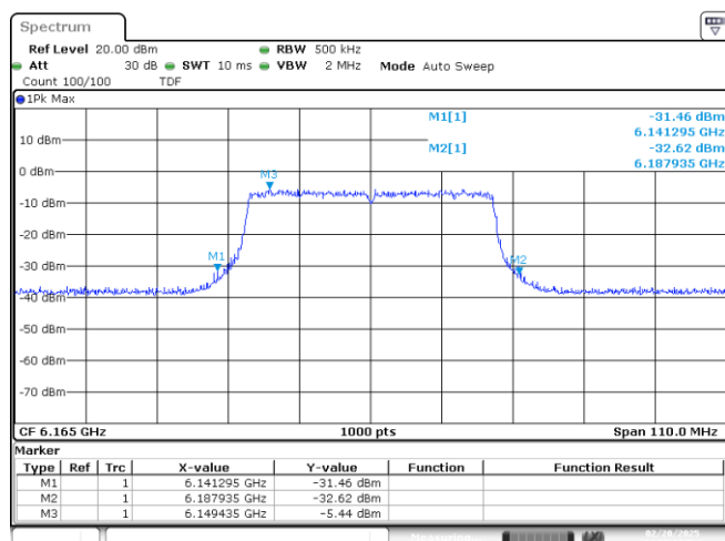
UNII-5 MIMO A 802.11ax/be40 ch43 6165MHz 26dB
