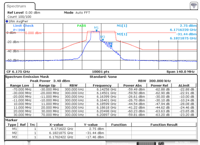
MIMO-A, 802.11ax/be20-MCS0, Ch45-6m-70
