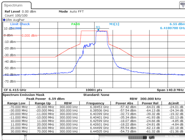
SISO-B, 802.11ax/be20-MCS0, Ch93-8m-53
