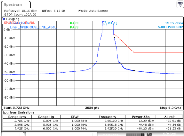
BE-NR-HIGH, SISO-A, 802.11a20-6Mbps, Ch177
