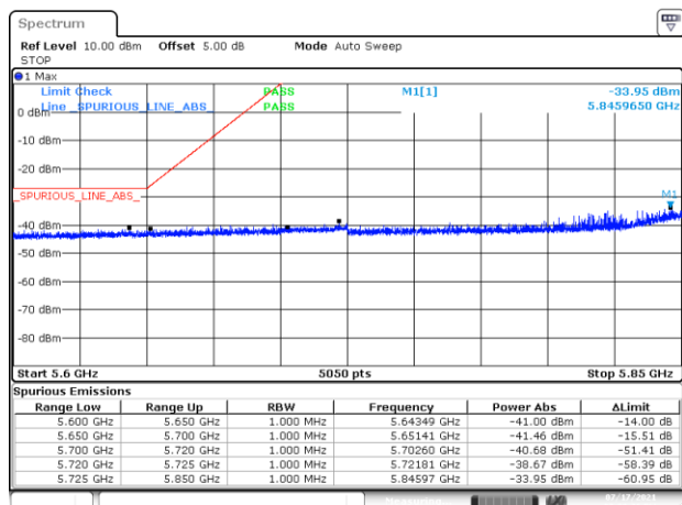
BE-NR-LOW, SISO-B, 802.11ax20-HE0, Ch177
