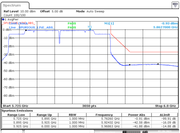
BE-NR-HIGH, MIMO-A, 802.11ax160-HE0, Ch163
