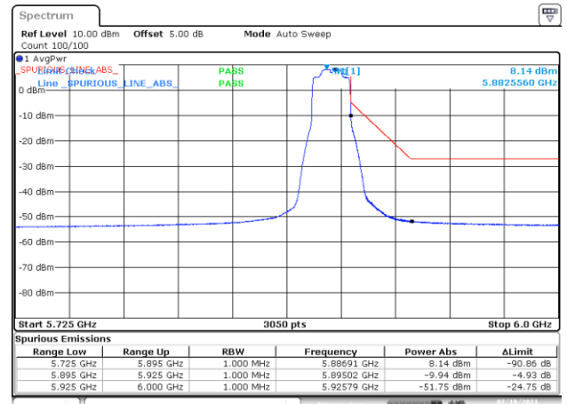
BE-NR-HIGH, MIMO-A, 802.11ax20-HE0, Ch177
