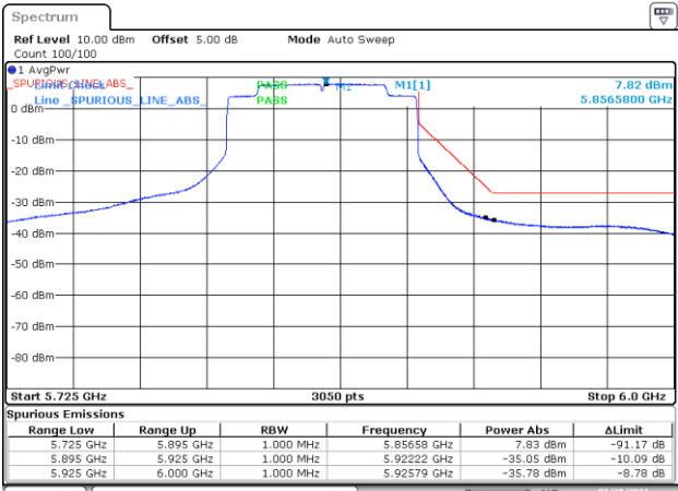
BE-NR-HIGH, MIMO-B, 802.11ax80-HE0, Ch171
