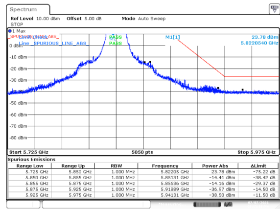
BE-NR-HIGH, SISO-A, 802.11a-6Mbps, Ch165
