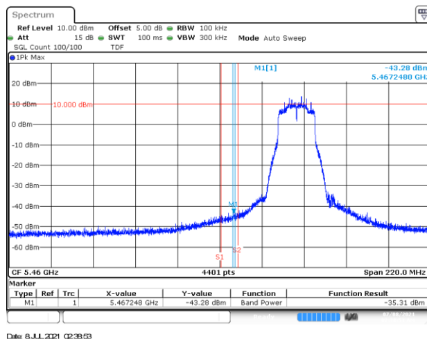
BE-NR-LOW, MIMO-A, 802.11ax20-HE0, Ch100
