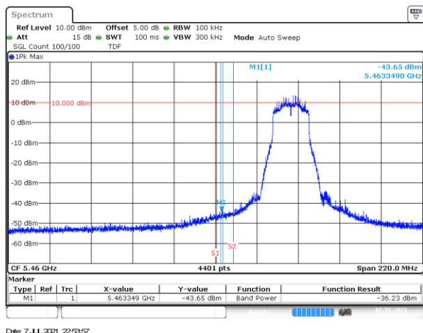
BE-R-LOW, MIMO-A, 802.11ax20-HE0, Ch100
