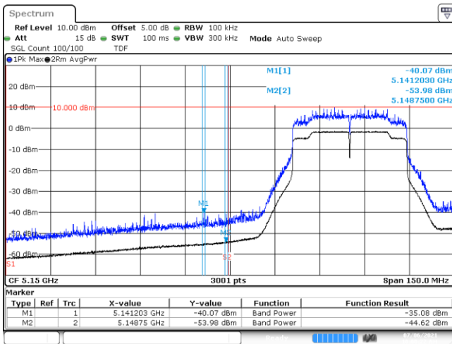
BE-R-LOW, SISO-A, 802.11ax40-HE0, Ch38
