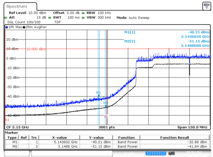
BE-R-LOW, SISO-A, 802.11ax80-HE0, Ch42
