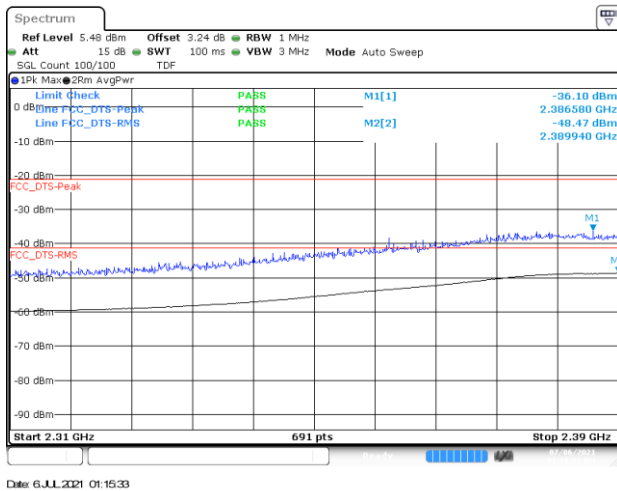
BE-R-LOW, MIMO-A, 802.11ax40-HE0, Ch3
