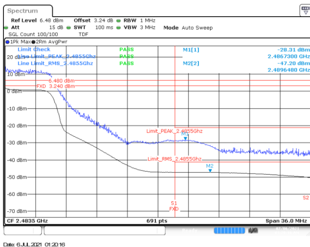
BE-R-HIGH, MIMO-A, 802.11ax40-HE0, Ch9
