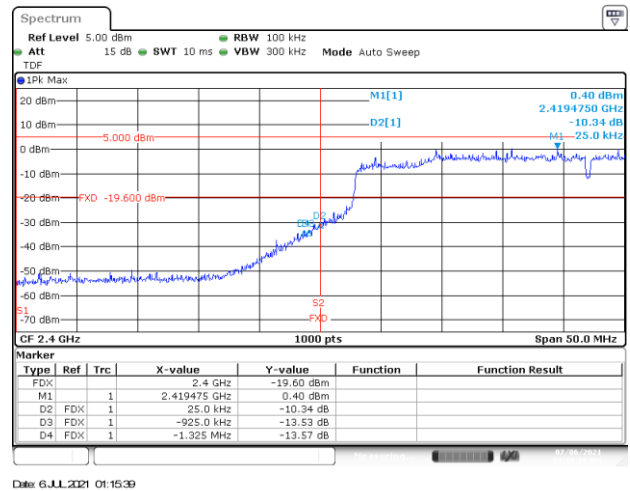
BE-NR, MIMO-A, 802.11ax40-HE0, Ch3
