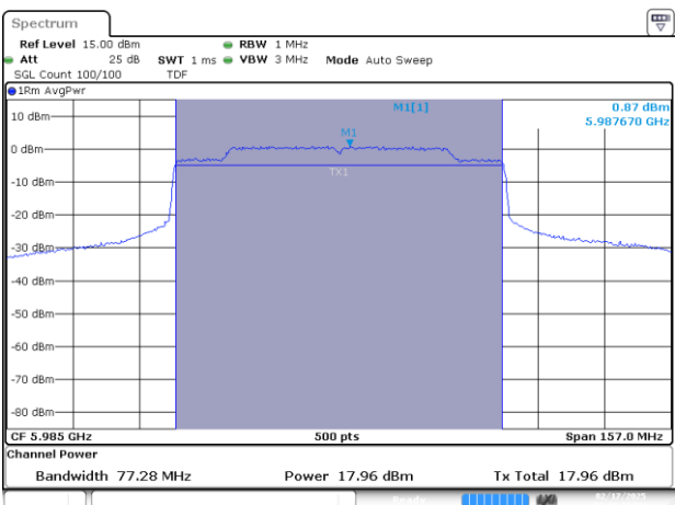
SISO A-802.11ax-80MHz-Ch7-5985MHz-MCS0
