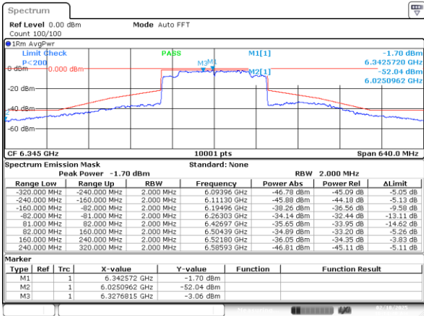
MIMO B-802.11ax-160MHz-Ch79-6345MHz-MCS0
