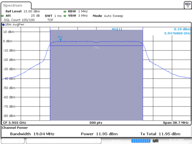
SISO A-802.11ax-20MHz-Ch1-5955MHz-MCS0
