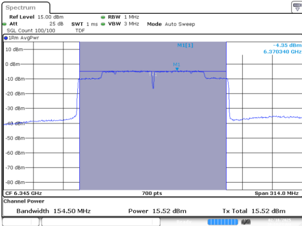
MIMO B-802.11ax-160MHz-Ch79-6345MHz-MCS0
