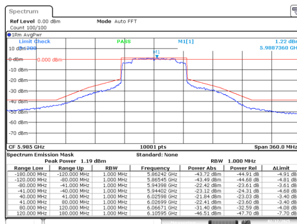
SISO A-802.11ax-80MHz-Ch7-5985MHz-MCS0
