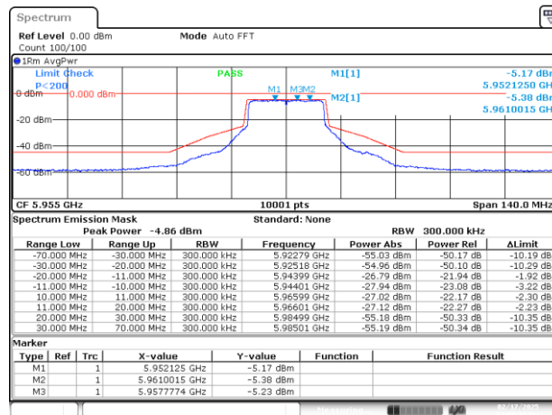
SISO A-802.11ax-20MHz-Ch1-5955MHz-MCS0
