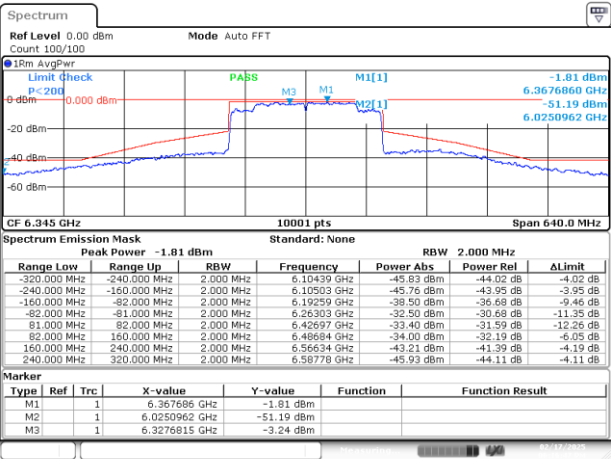
MIMO A-802.11ax-160MHz-Ch79-6345MHz-MCS0
