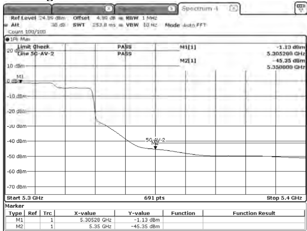
ax160-5250-996-S67-AV-SISO B-RU
