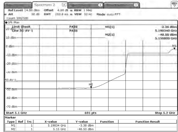
ax160-5250-1-AV-SISO A
