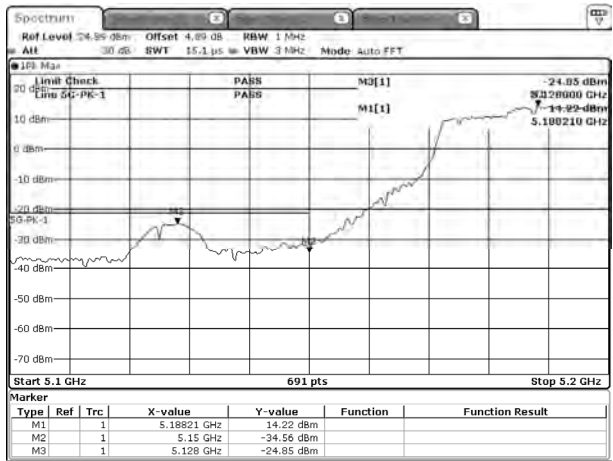
ac80-5210-SISO A-PK
