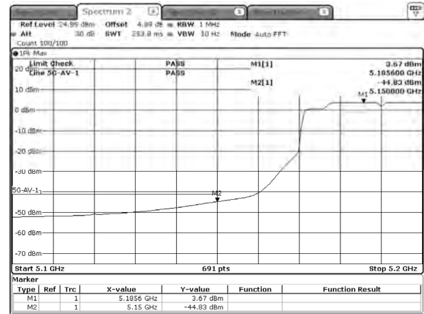
ax40-5190-SISO B-AV
