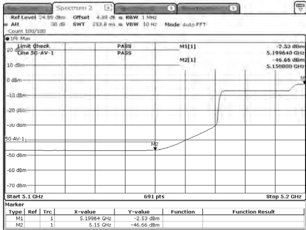
ac160-5250-1-SISO A-AV
