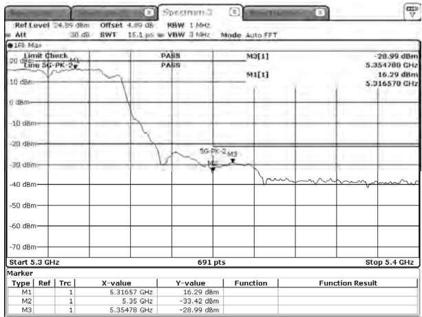
n40-5310-SISO A-PK
