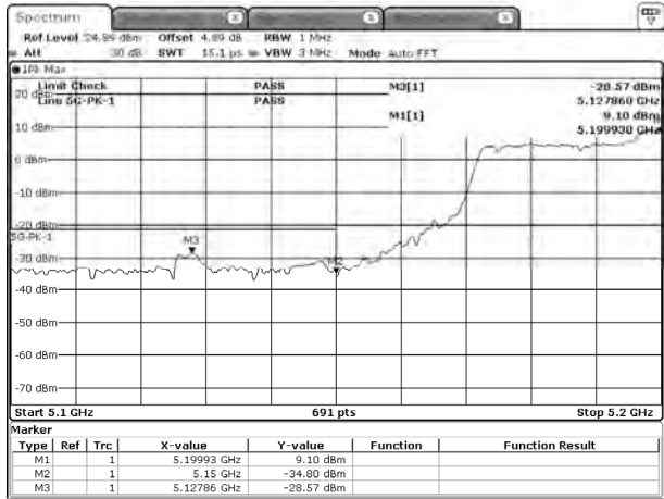
ac160-5250-1-SISO A-PK
