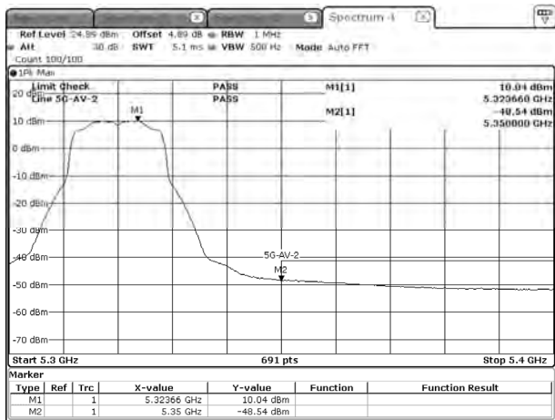
a-5320-SISO B-AV
