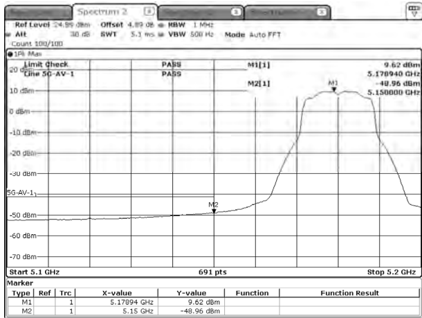
a-5180-SISO B-AV
