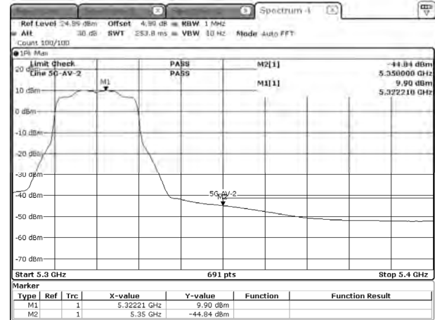
ax20-5320-AV-SISO A
