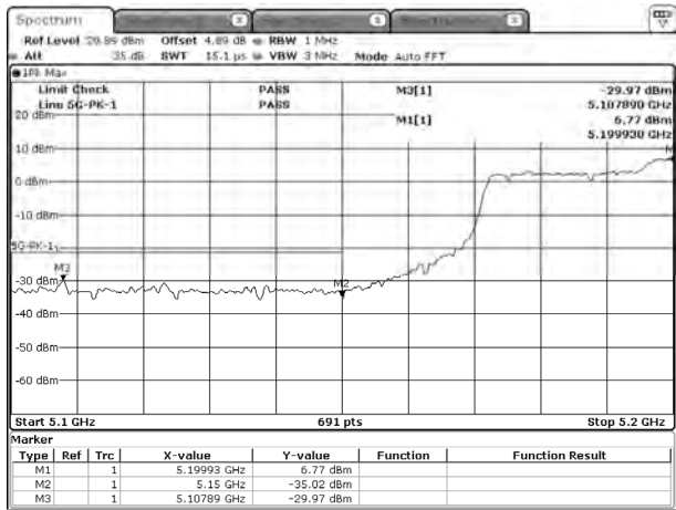
ac160-5250-1-PK-SISO B
