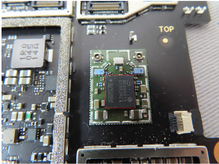
WiFi/BT Module
