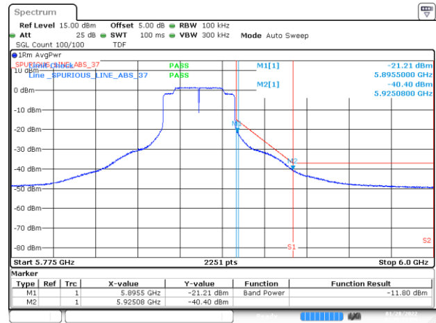
BE-NR-HIGH, SISO-B, 802.11ax40-HE0, Ch175
