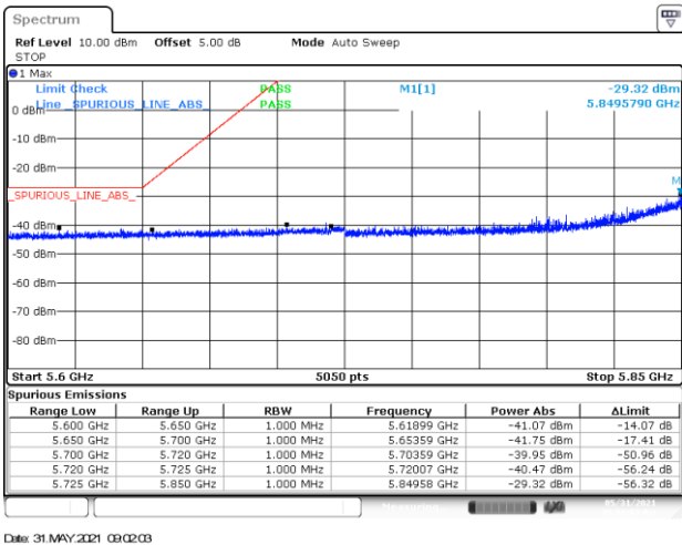
BE-NR-LOW, SISO-B, 802.11ax20-HE0, Ch177
