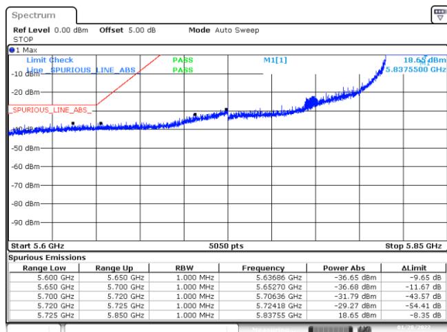
BE-NR-LOW, MIMO-A, 802.11ax80-HE0, Ch171
