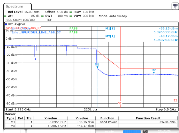
BE-NR-HIGH, SISO-A, 802.11ax160-HE0, Ch163
