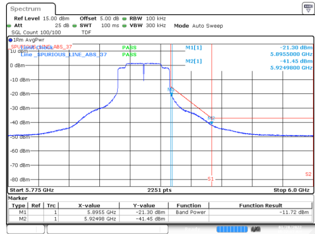
BE-NR-HIGH, SISO-A, 802.11ax40-HE0, Ch175
