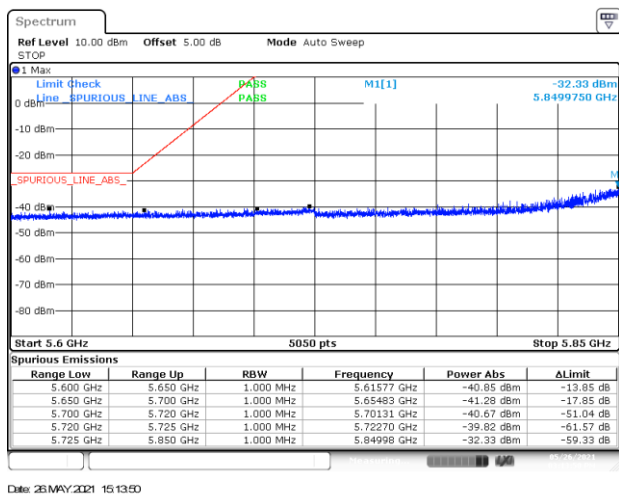
BE-NR-LOW, SISO-A, 802.11a20-6Mbps, Ch177
