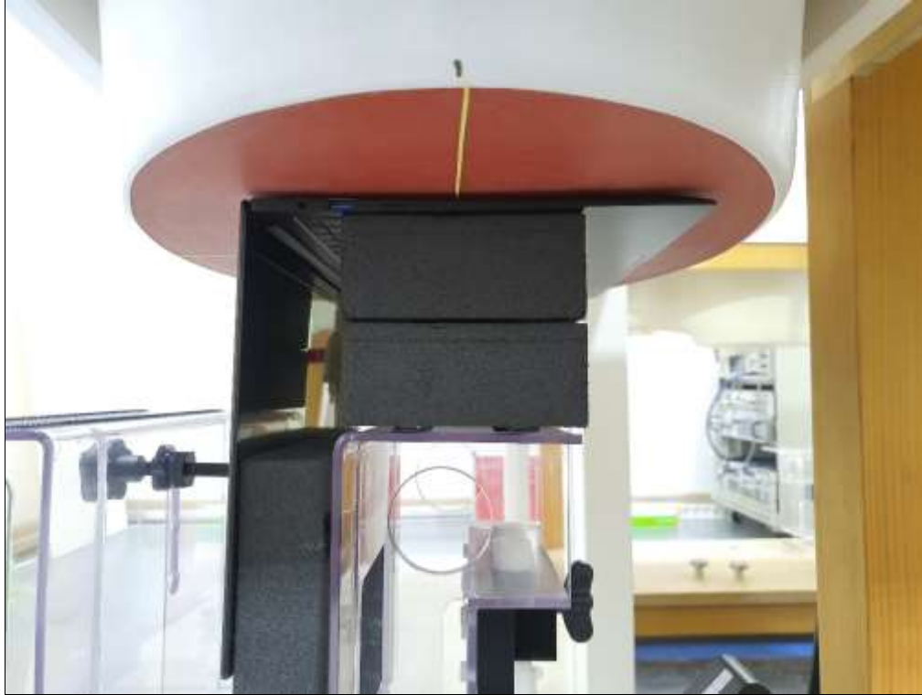
E.1) Body_SAR Rear(0 mm)
